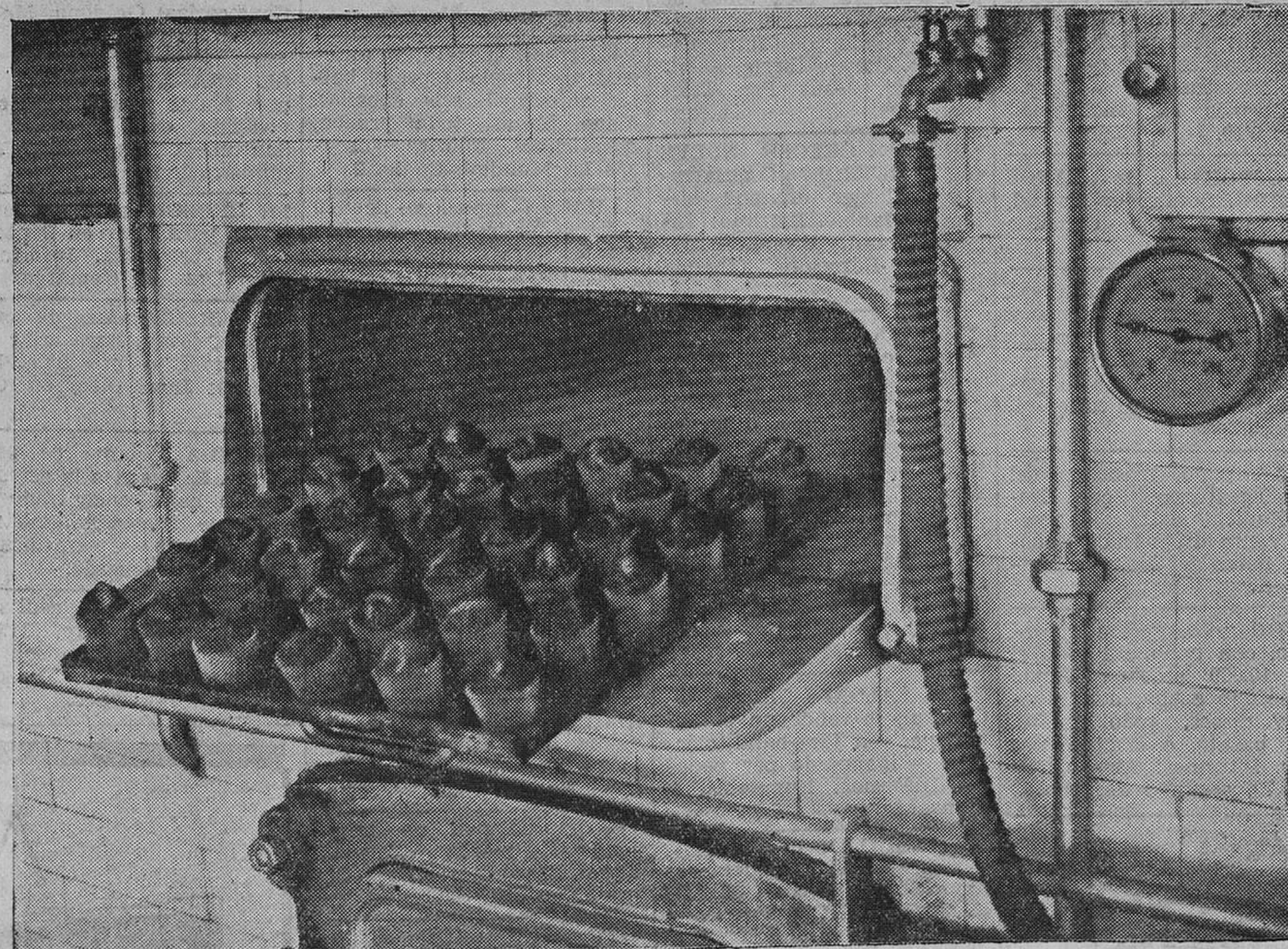
Fronte del horno, tipo eclético, construido por don Francisco Guesalaga, de San Sebastián.
