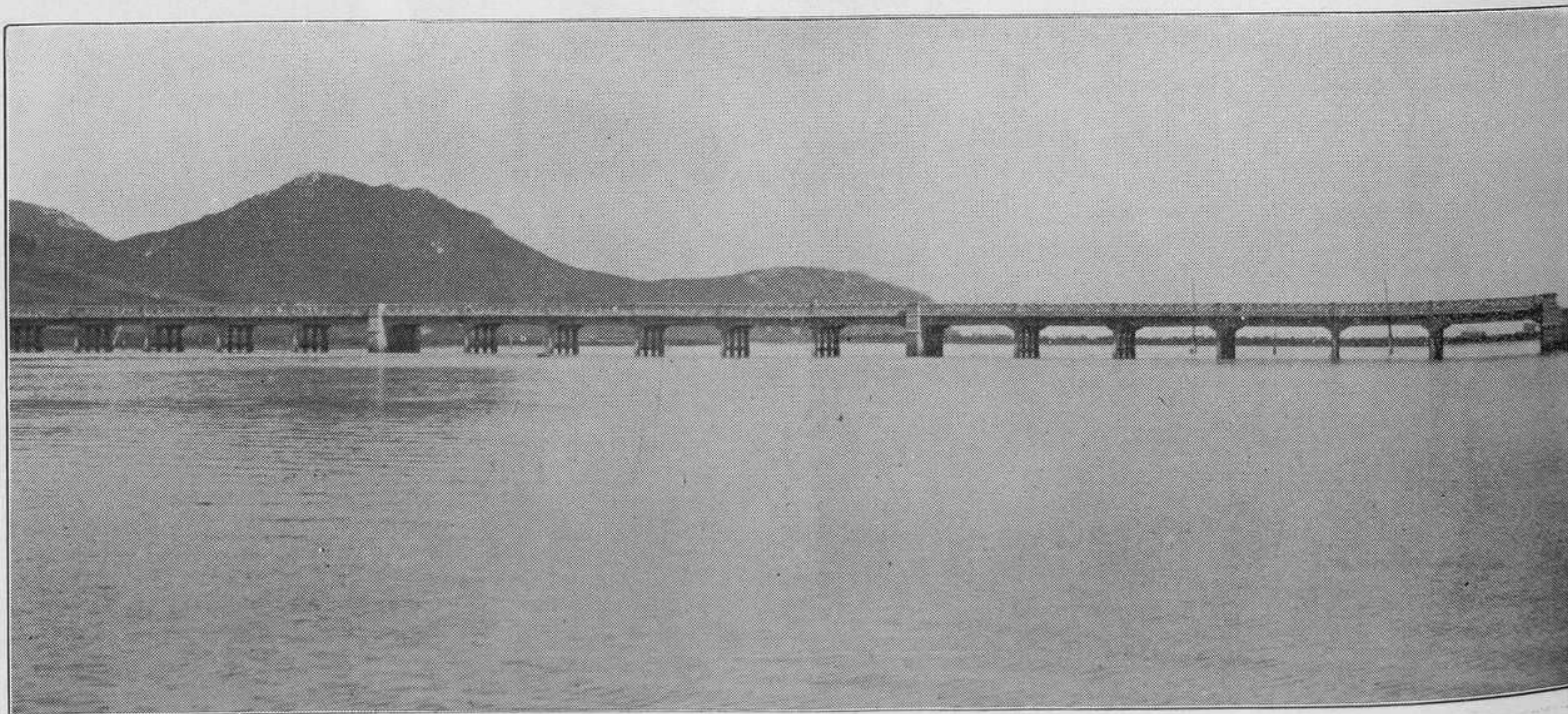
Uno de los tres grandes puentes recientemente construidos en la nueva carretera que une a Santoña con el pueblo de Cicero.
