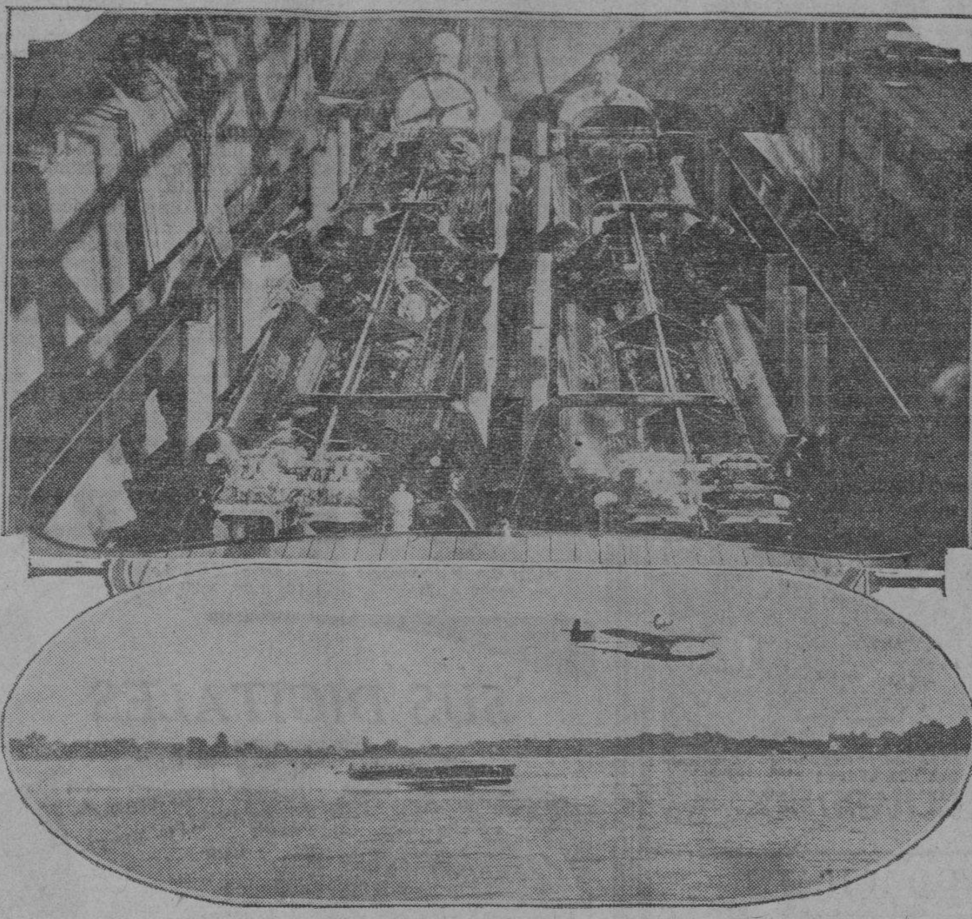
Arriba los cuatro motores Packard instalados en el "Miss America X" para contender con "Miss England III" en el Lago de St. Clair dentro de poco y luchar por la copa Harmsworth. En estas carreras se disputará una vez más la supremacía en botes de motor. "Miss England III" que aparece abajo corriendo a la par que un aeroplano, será guiado por Kaye Don, mientras que "Miss America X" será guiado por Gar Wood.
