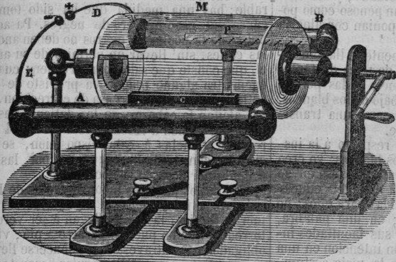
FIG. 1.ª Máquina eléctrica de Nairne.
