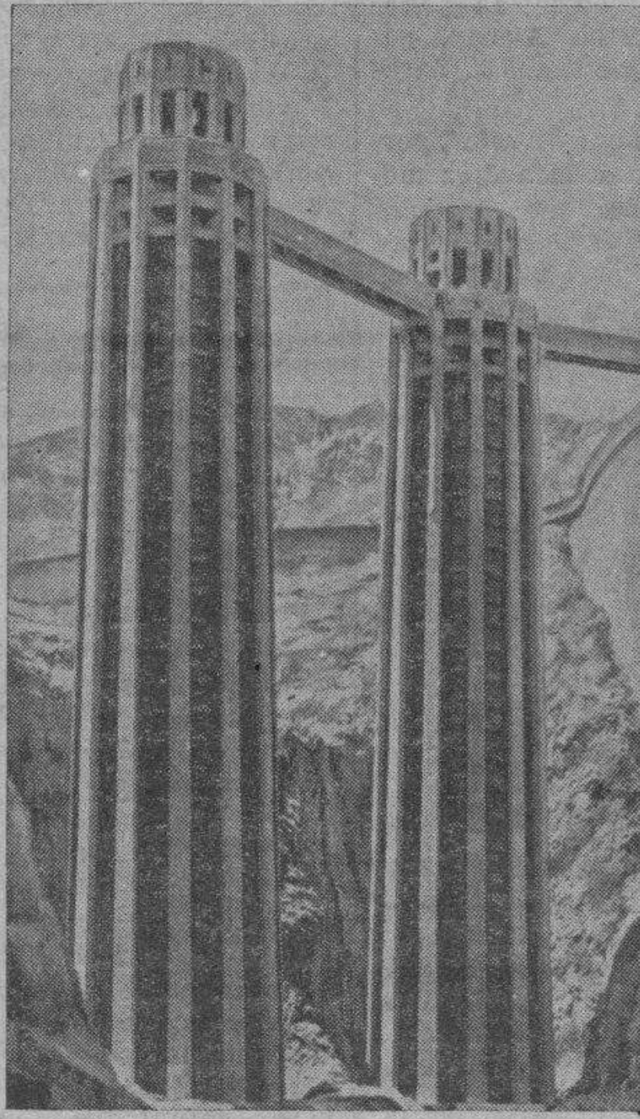
Maravillas técnicas. Dos torres de noventa metros que han de realizar el control del dique de Boulder (U. S. A.) y que en caso de exceso facilitarán el desagüe por el acueducto de comunicación...
