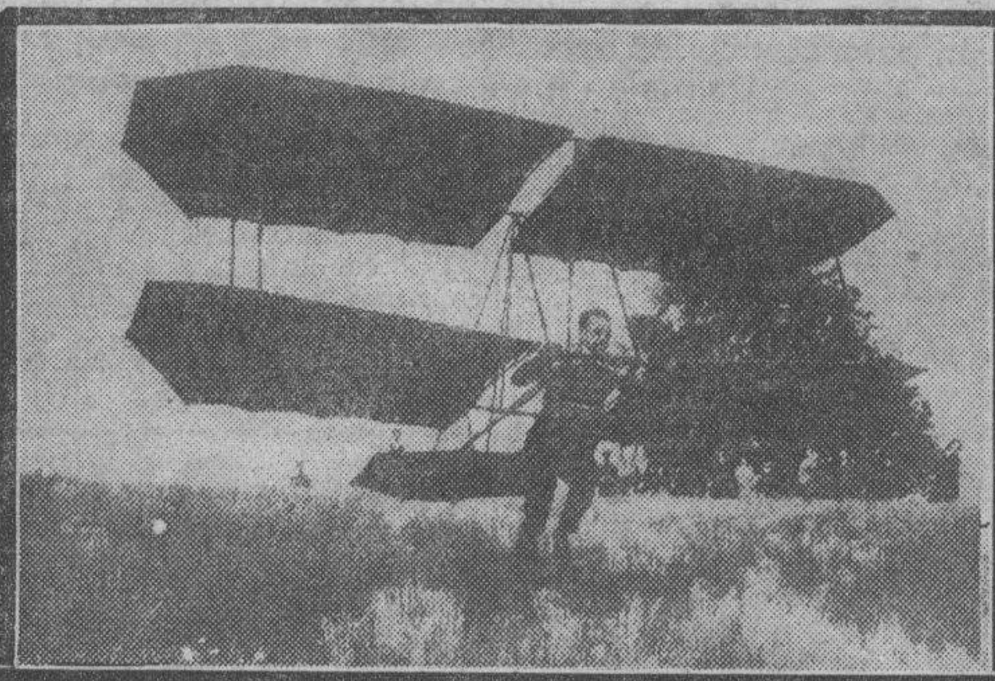
Hacia el avión de bolsillo. Este planeador, construido por el piloto alemán Hans Richter, cuesta sólo 175 reichmark; tiene cinco metros de envergadura, y pesa 28 libras alemanas. Puede empaquetarse y transportarse como equipaje. Su manejo no requiere aprendizaje.
