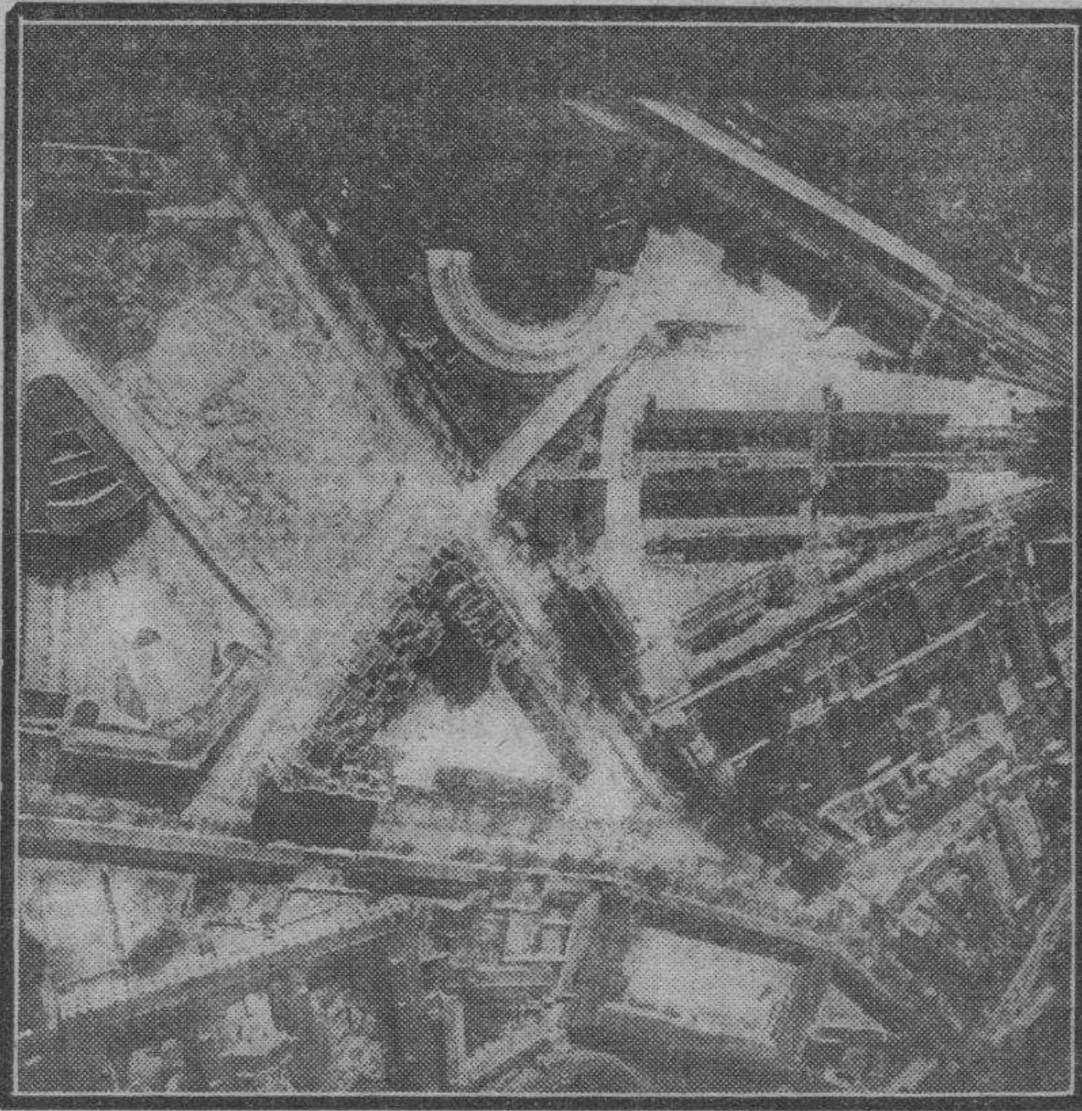
ZARAGOZA. — Estación de Madrid, Pabellones Militares y Casa-Refugio. Fotografía tomada por el Servicio de Fotogrametría Aérea.
