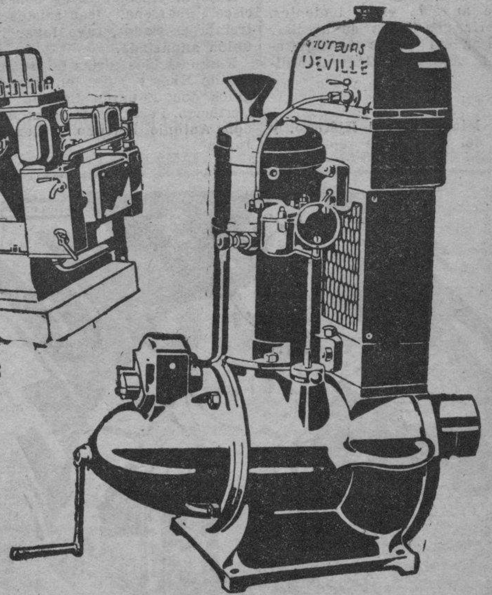
Motores a gasolina "DEVILLE" con radiador
