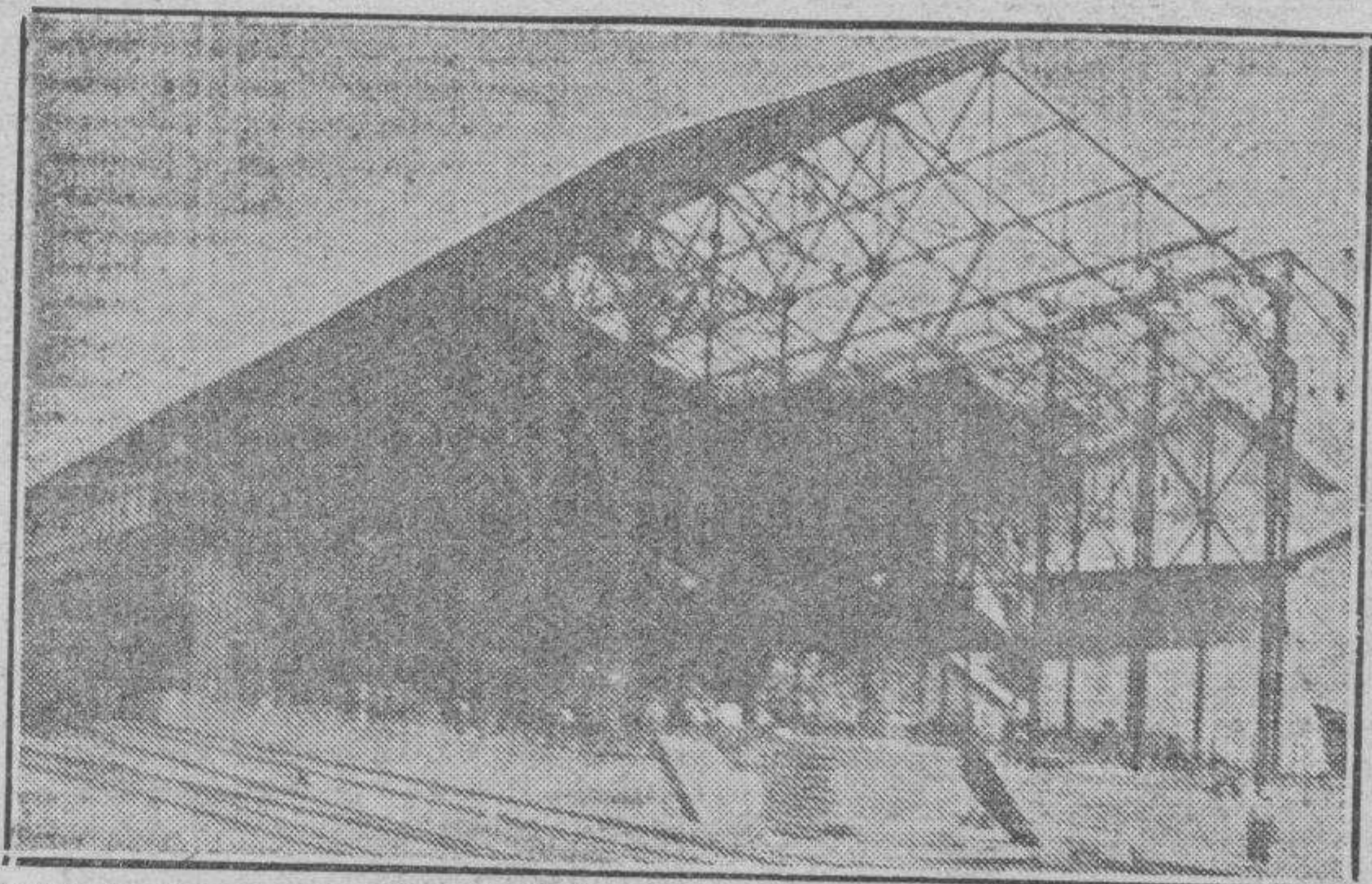
Almacén de superfosfatos de la Industrial Química, cuya formidable estructura metálica es obra de “Zaragoza Industrial”, S. A.
