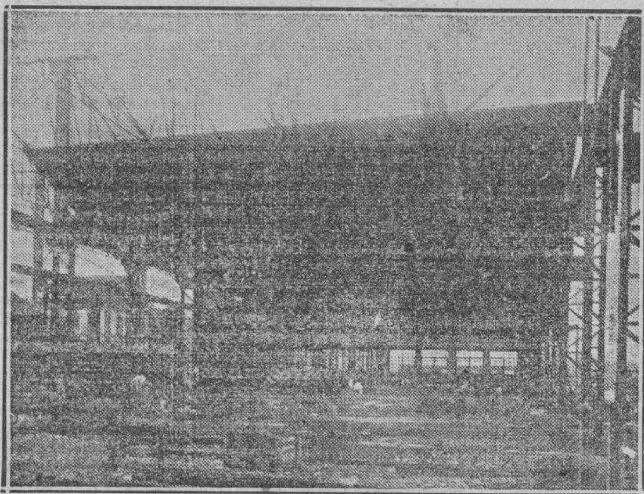
Los antiguos talleres de Cardé y Escoriaza han levantado estas colosales naves metálicas, que son obra igualmente de “Zaragoza Industrial”. S. A.
