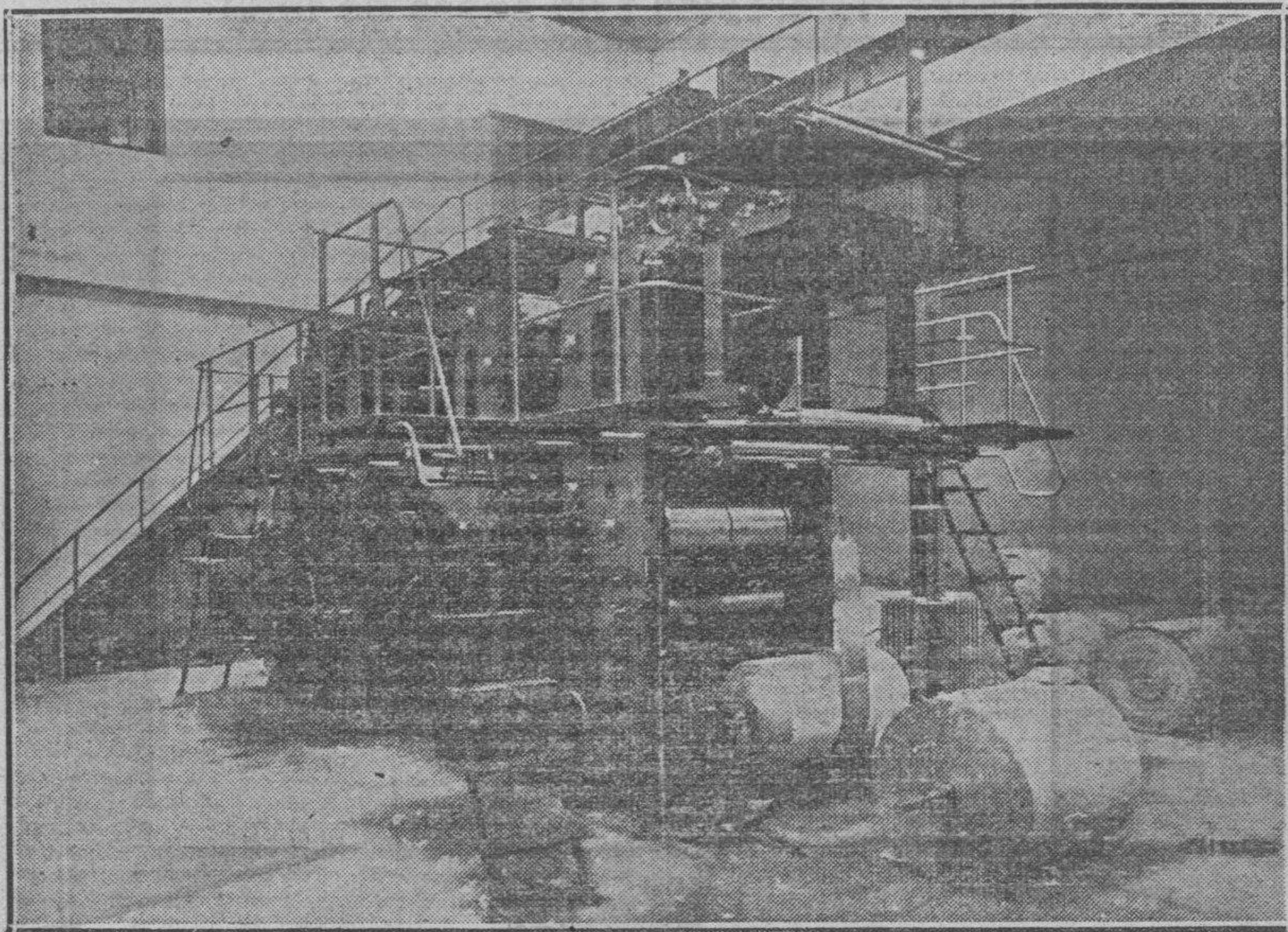
La nueva rotativa en la que, desde hoy, se imprime LA VOZ DE ARAGON. Se trata de una máquina capaz de tirar número s hasta de 32 páginas, y de un tiraje de 24,000 ejemplares a la hora.
