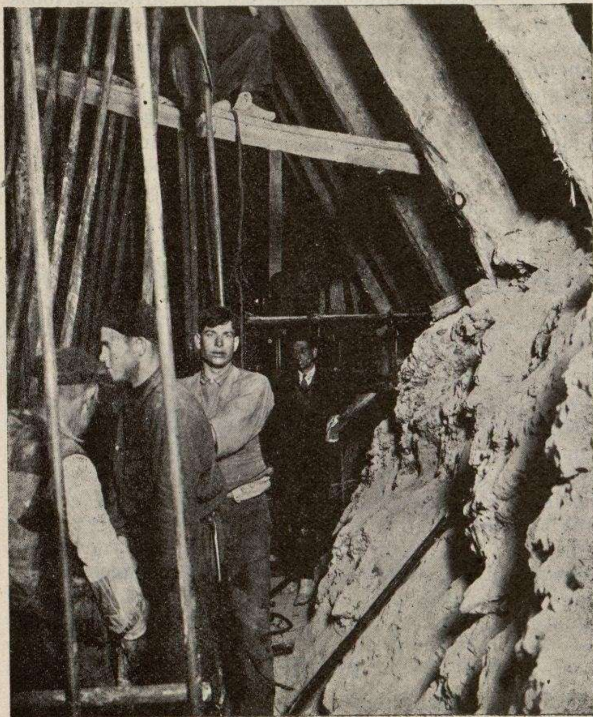
FERROCARRIL DE LÉRIDA A ST. GIRONS.—Interior del túnel. Detalle de la entibación y armadura de hierro
