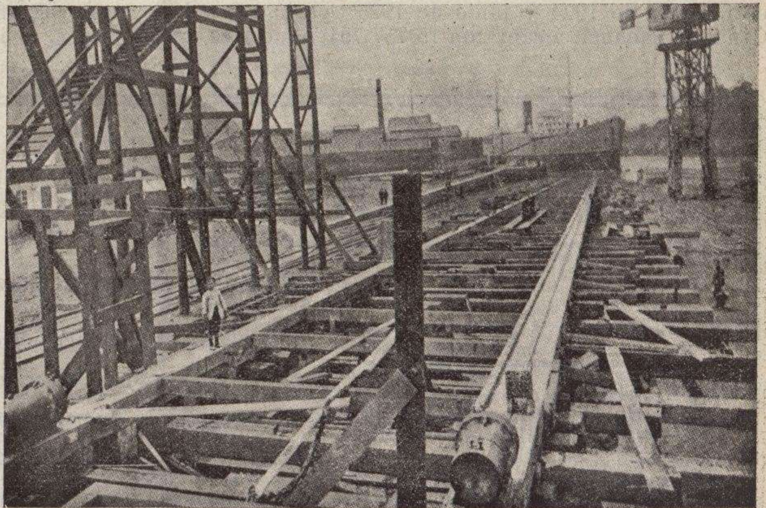
Grada de los astilleros "Euskalduna"
