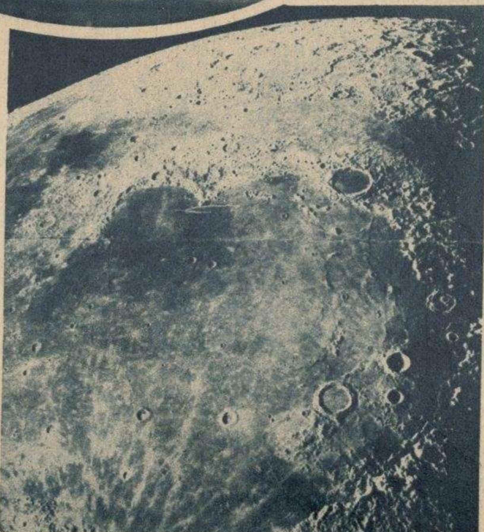
Cuadrante nordeste de la Luna. Región del mar de las lluvias. Magnífica fotografía obtenida en el Observatorio de Mt. Wilson, California, con el gran reflector "Hooker," de 101 pulgadas de diámetro actualmente el mayor del mundo, por el profesor Francis G. Pease.
