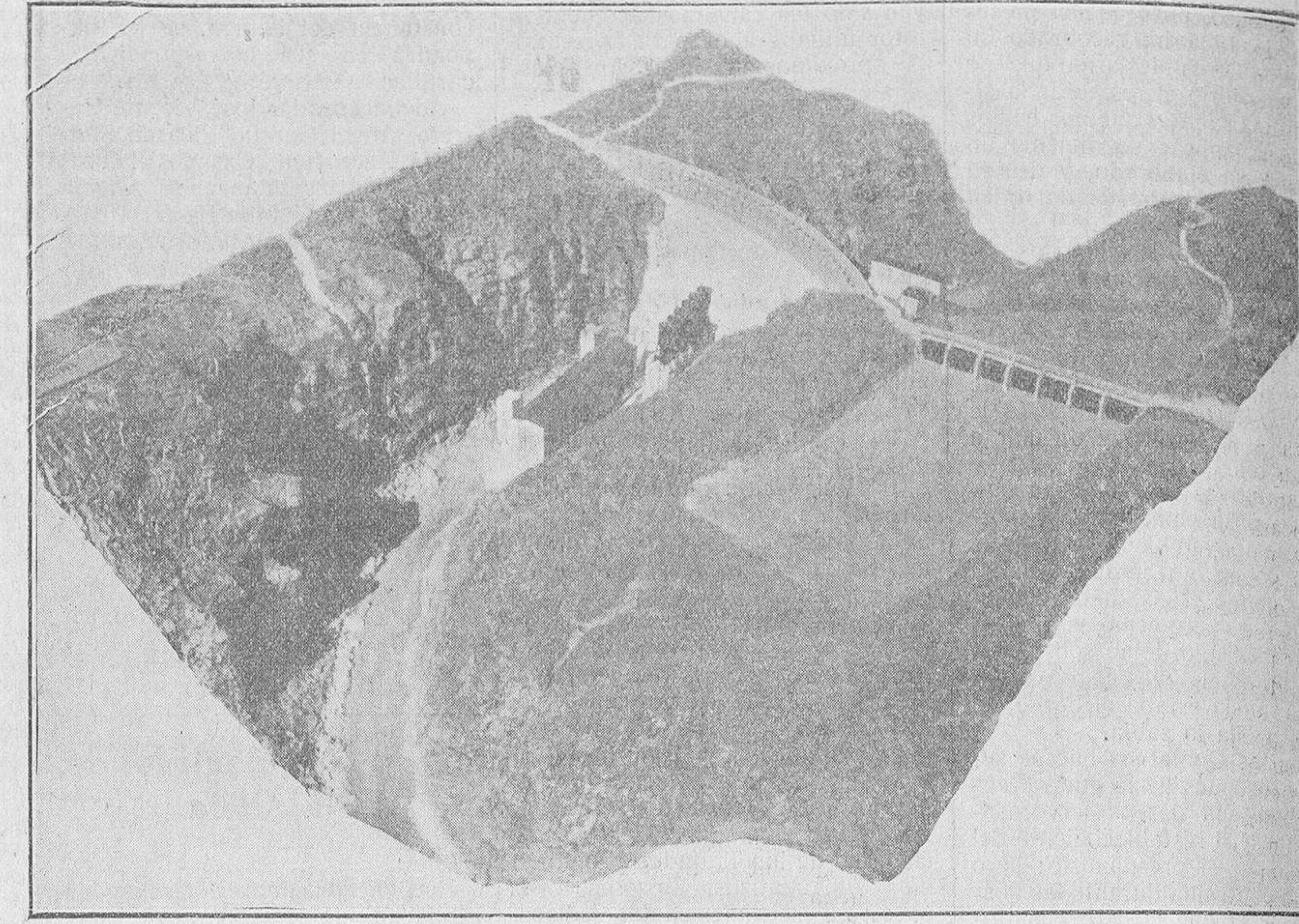
Maqueta del salto de cien mil caballos en Ricobayo (Zamora), que pronto comenzará a construirse.
