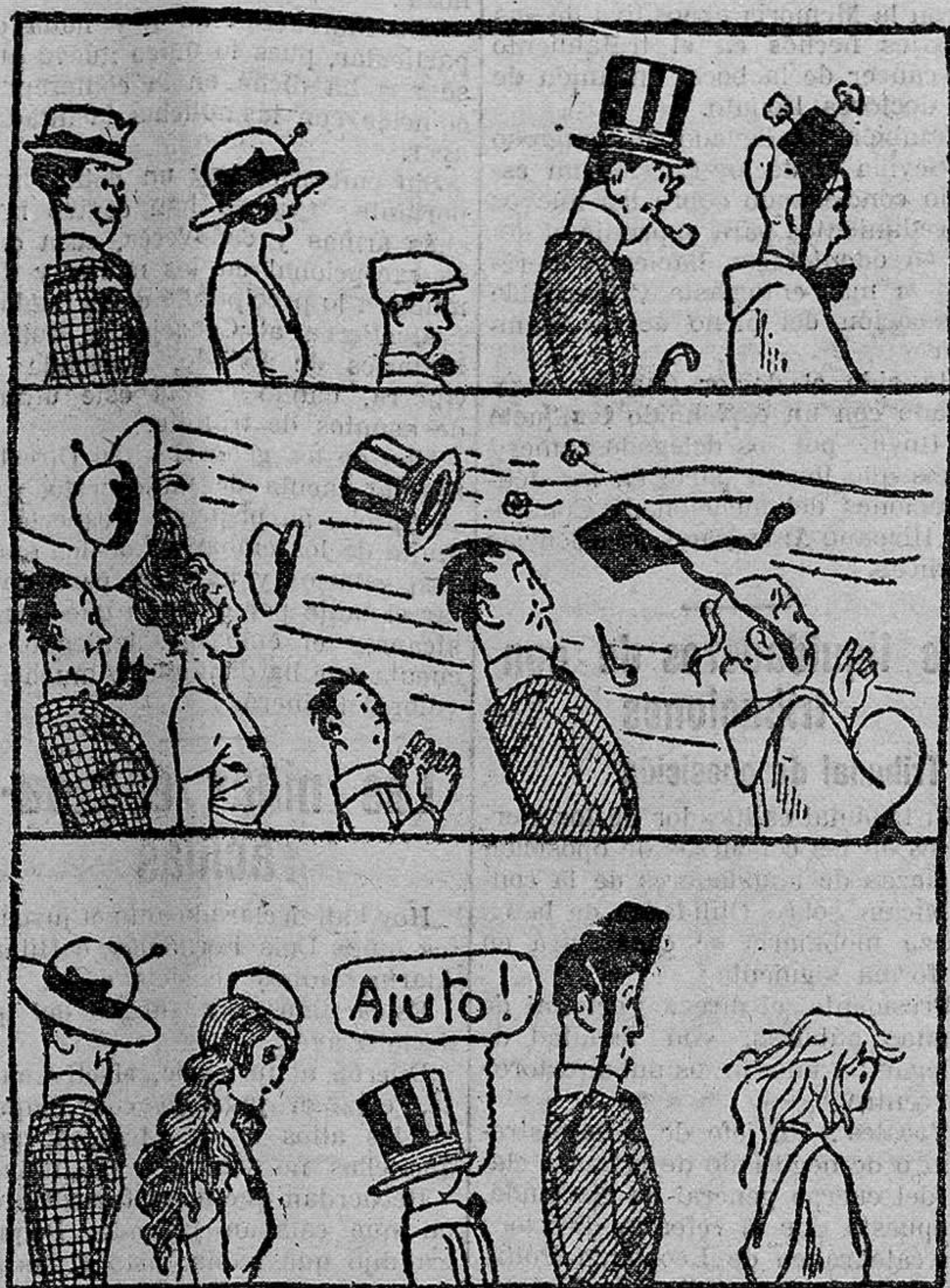
Transformaciones instantaneas
