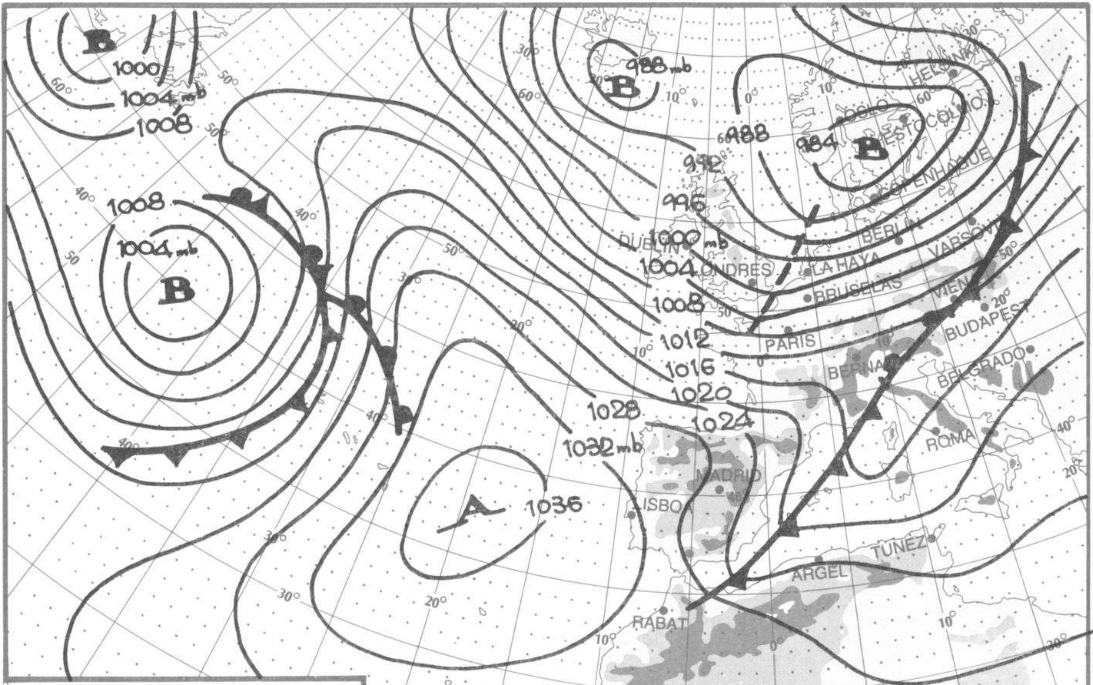
ANÁLISIS EN SUPERFICIE a 12 h (TMG) Día 26/12/1997.....
