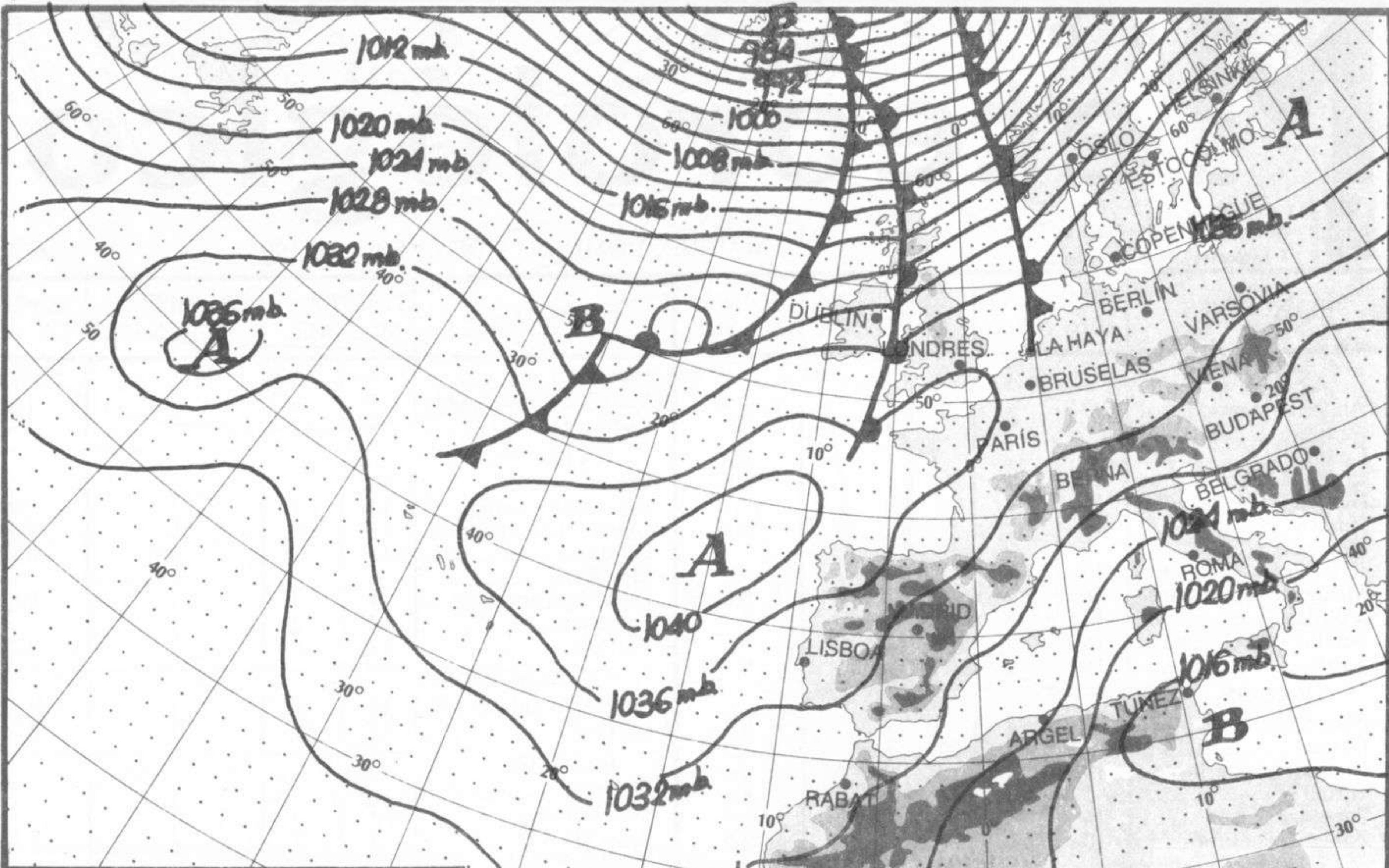
ANÁLISIS EN SUPERFICIE a 12 h (TMG) Día 07/01/1995
