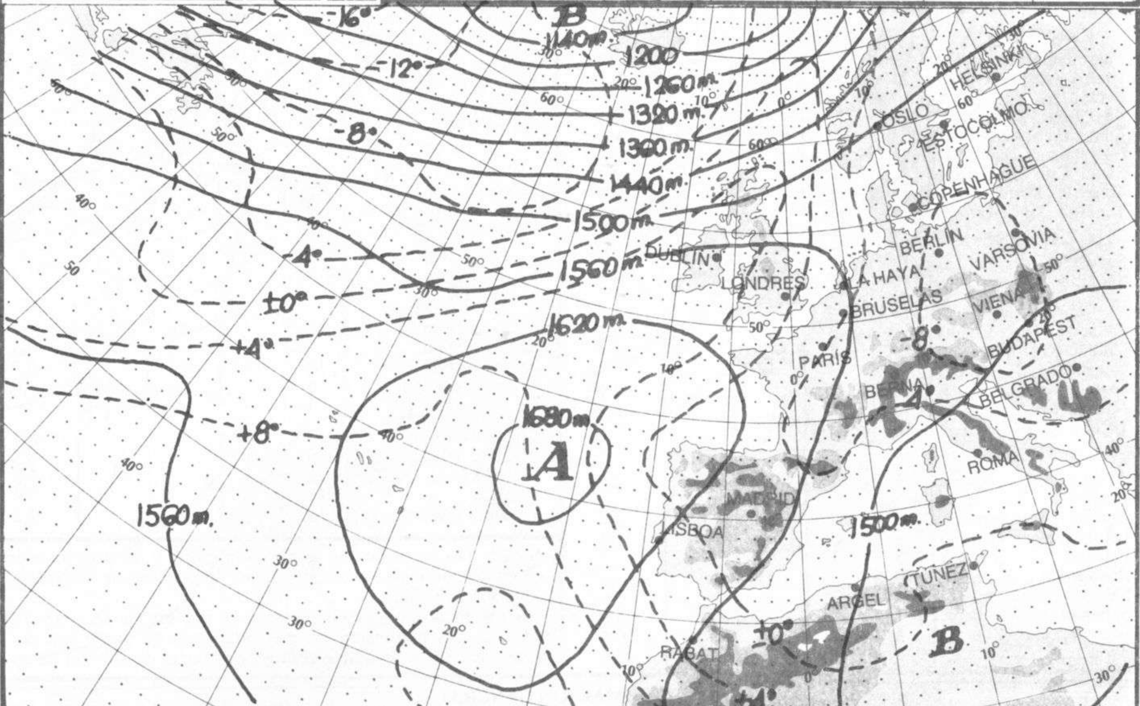
TOPOGRAFÍA DE LA SUPERFICIE DE 850 hPa a 12 h (TMG) Día 07/01/1995
