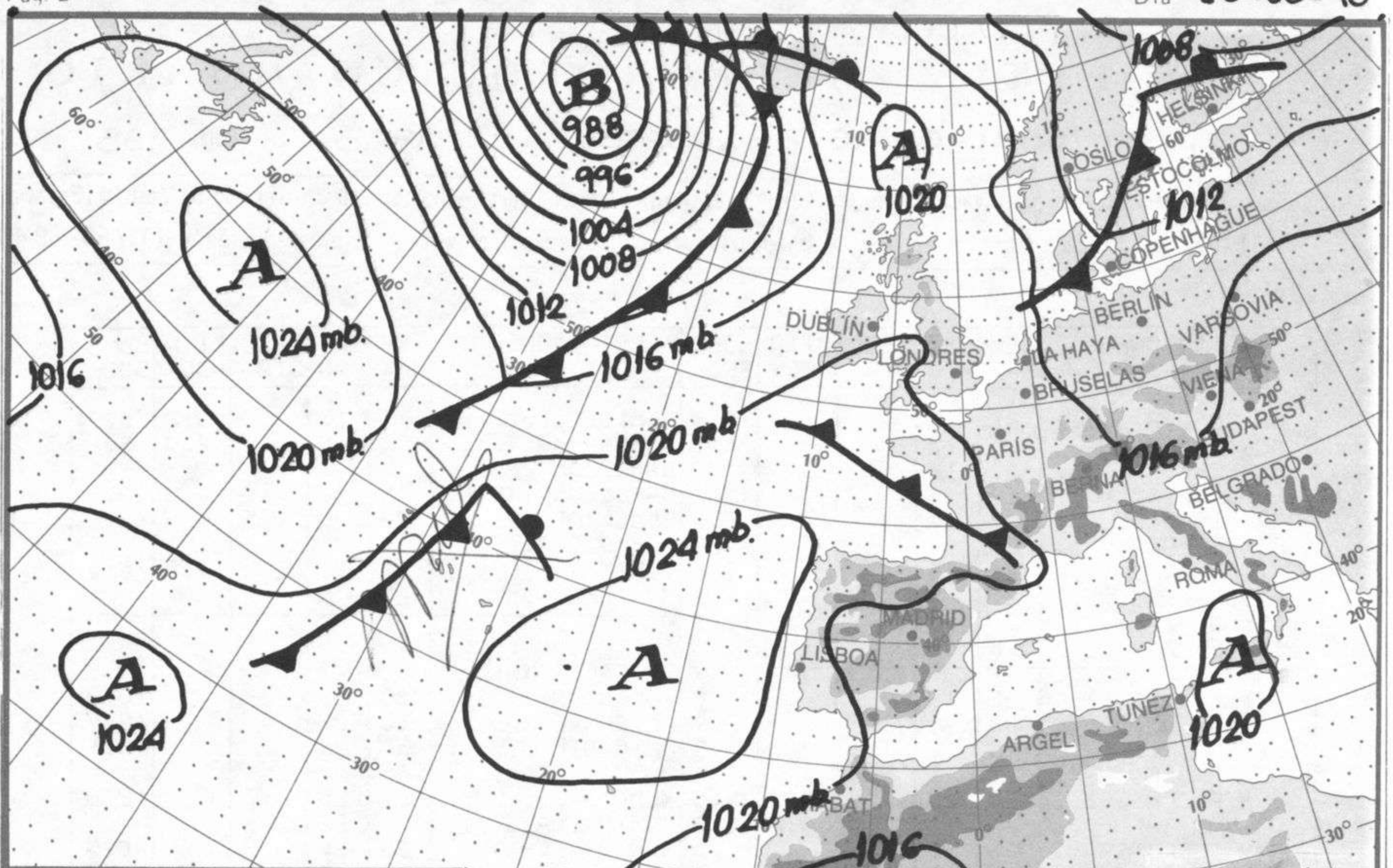
ANALISIS EN SUPERFICIE a 12 h. (TMG) Día 25-08-90
