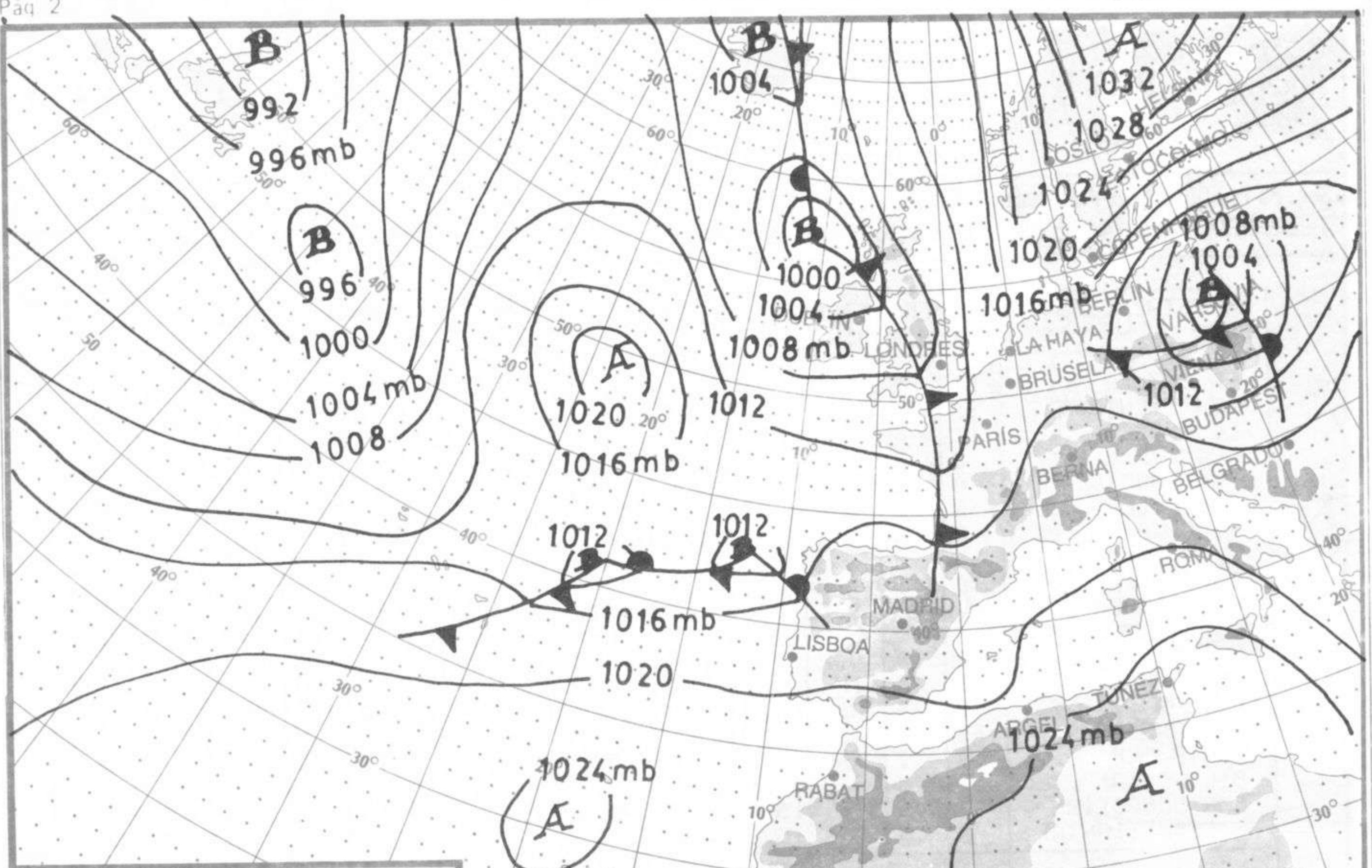
ANALISIS EN SUPERFICIE a 12 h. (TMG) Día 9-1-87
