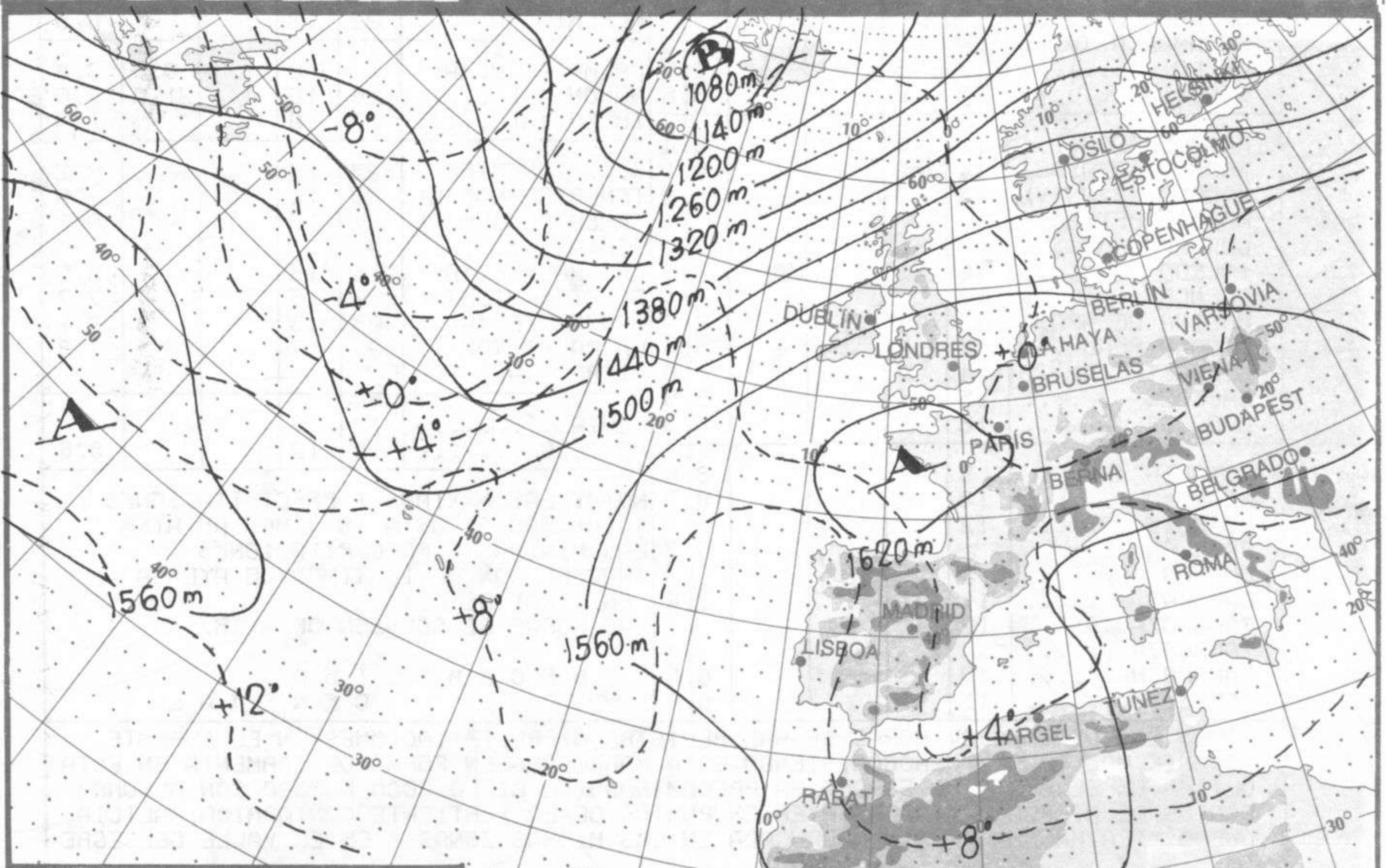
TOPOGRAFIA DE LA SUPERFICIE DE 850 hPa
