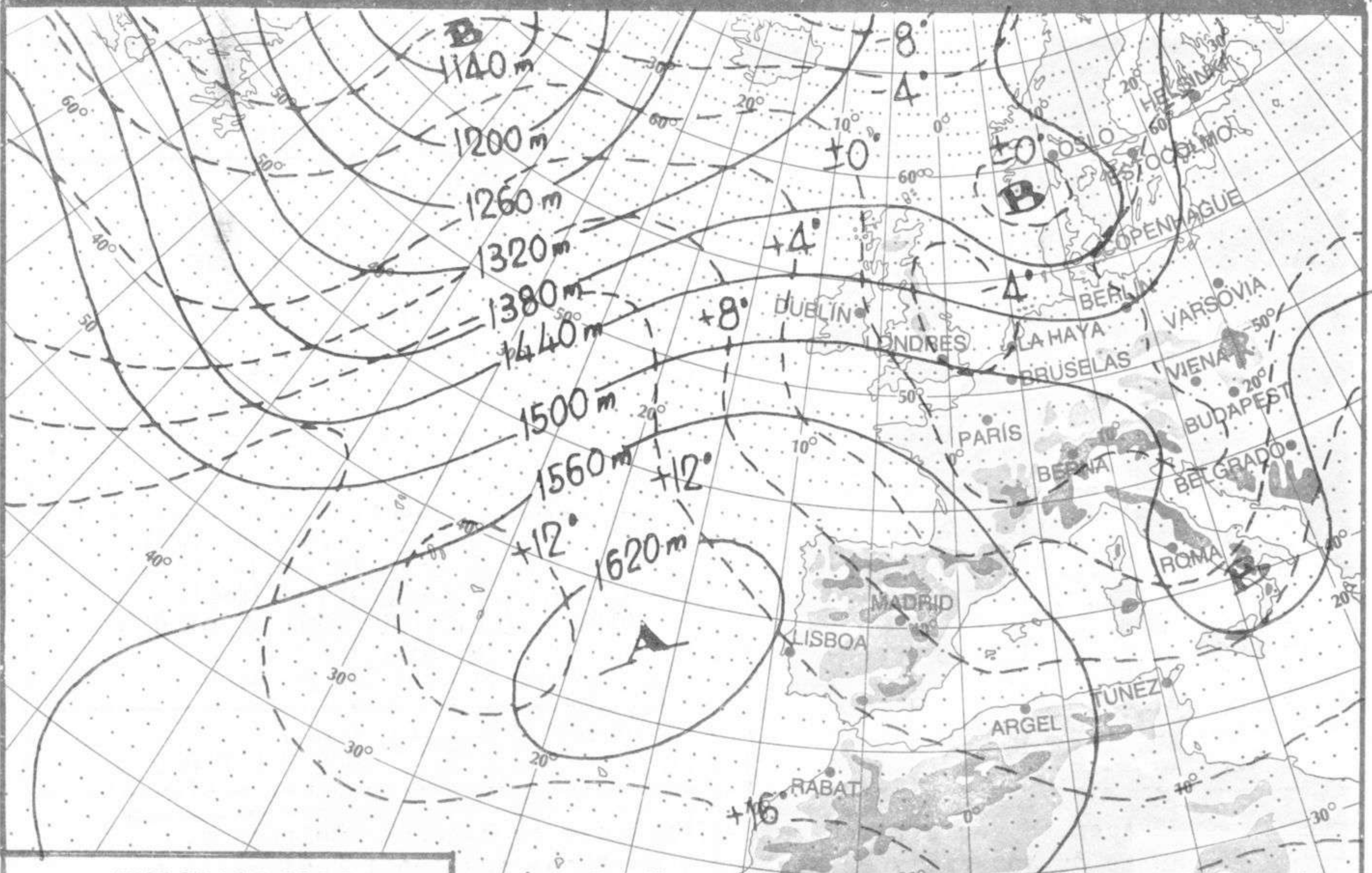
TOPOGRAFIA DE LA SUPERFICIE DE 850 HPa a 12 h. (TMG) Día ..... 26-10-86 .....
