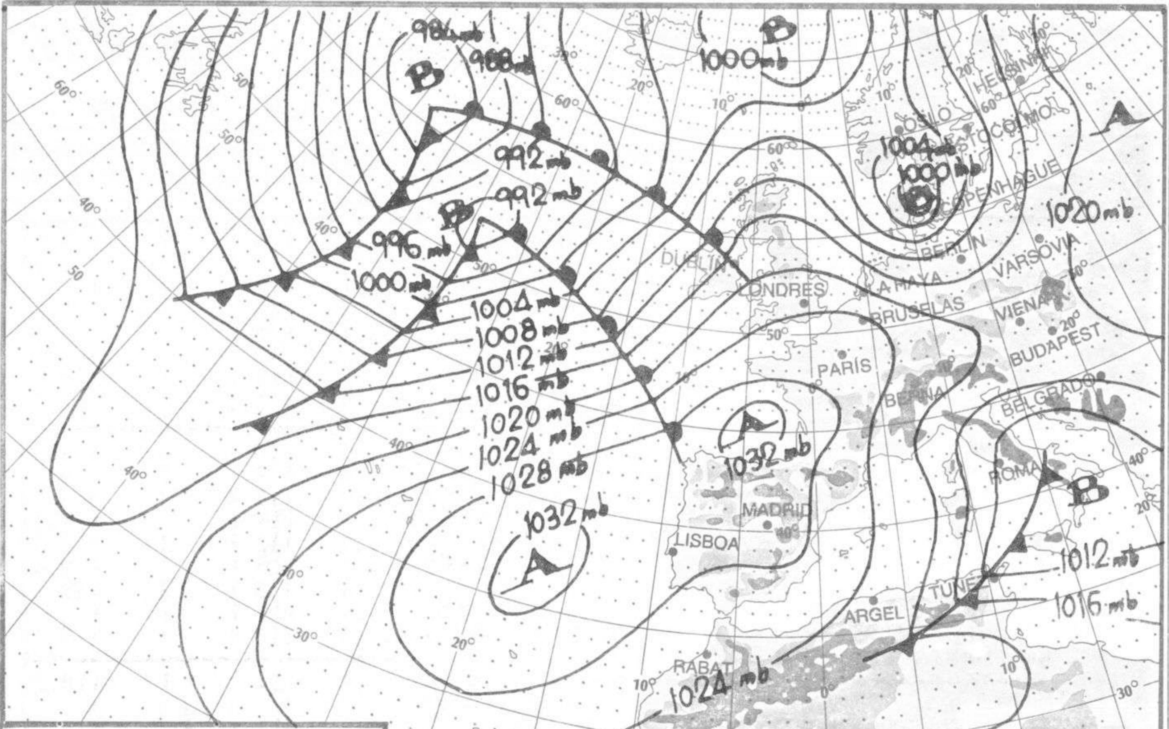
ANALISIS EN SUPERFICIE a 12 h. (TMG) Día ..... 26-10-86 .....
