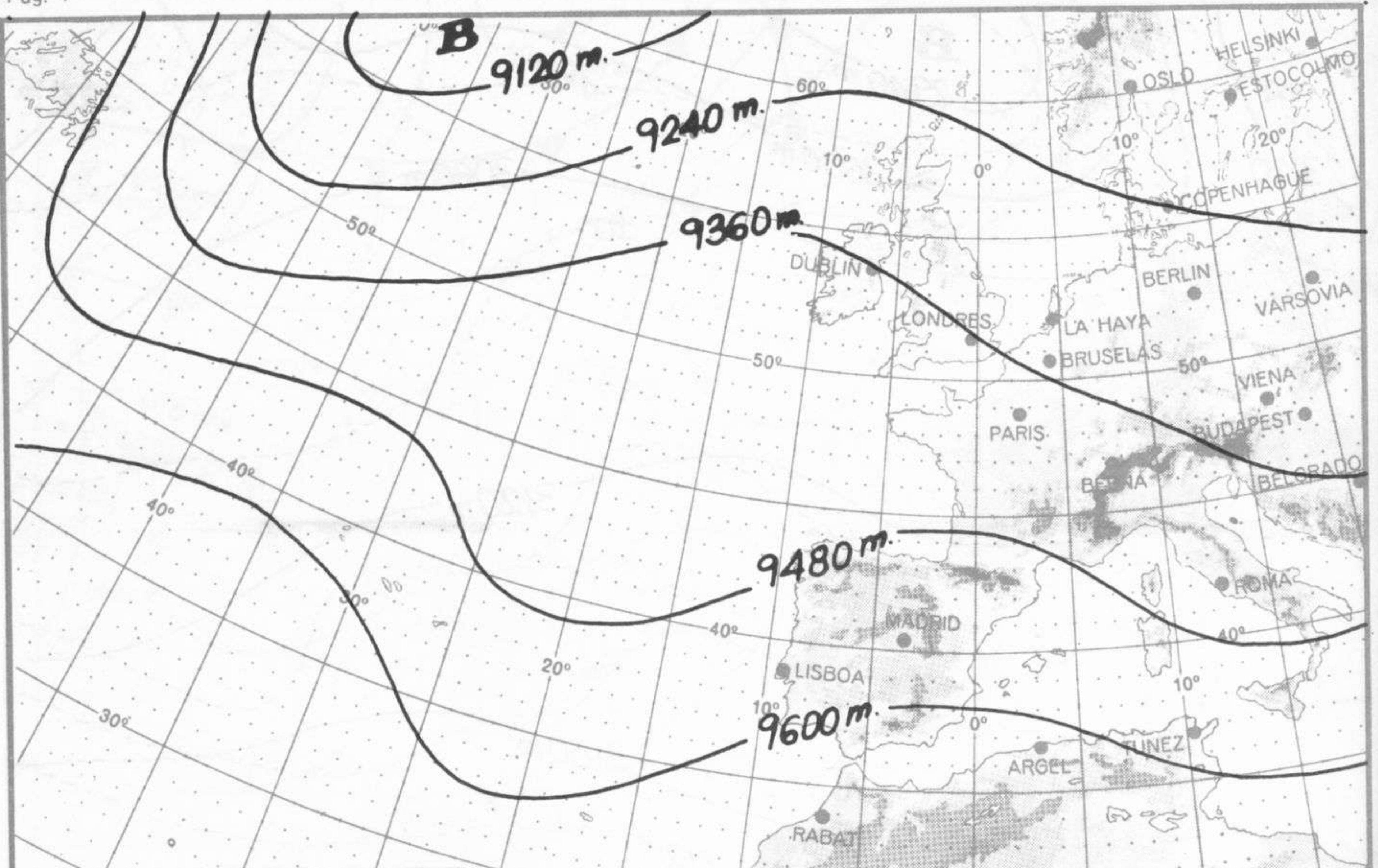
TOPOGRAFIA DE LA SUPERFICIE DE 300 mb. a 12 h. (TMG) Día 15-8-84.
