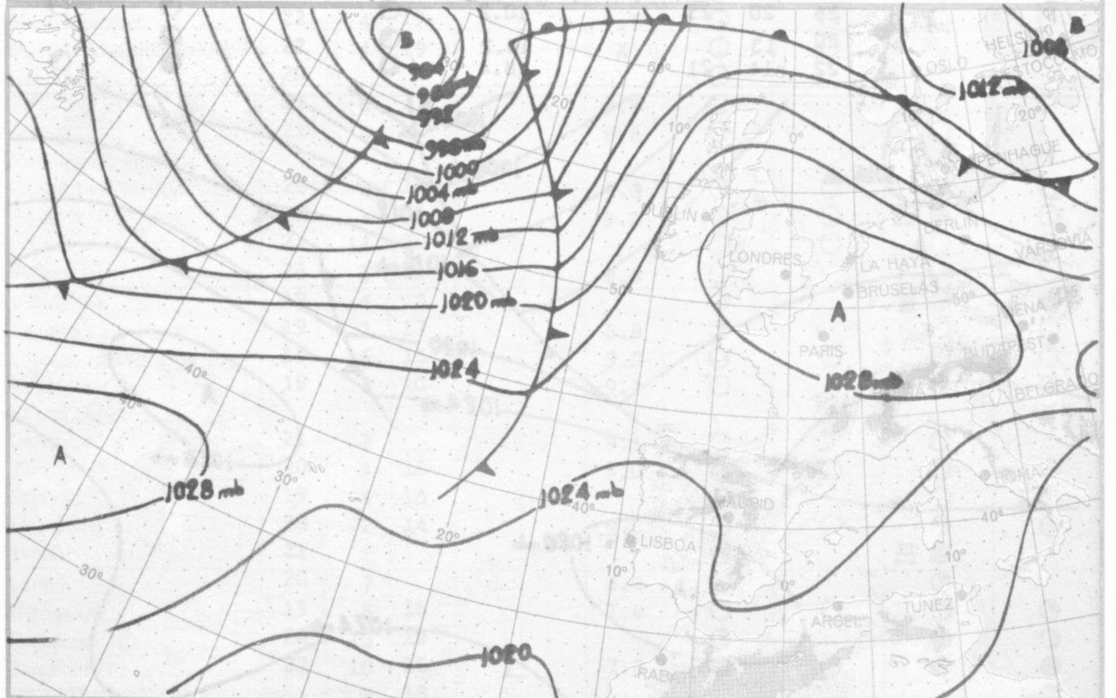
ANALISIS EN SUPERFICIE a 0 h.(TMG)
