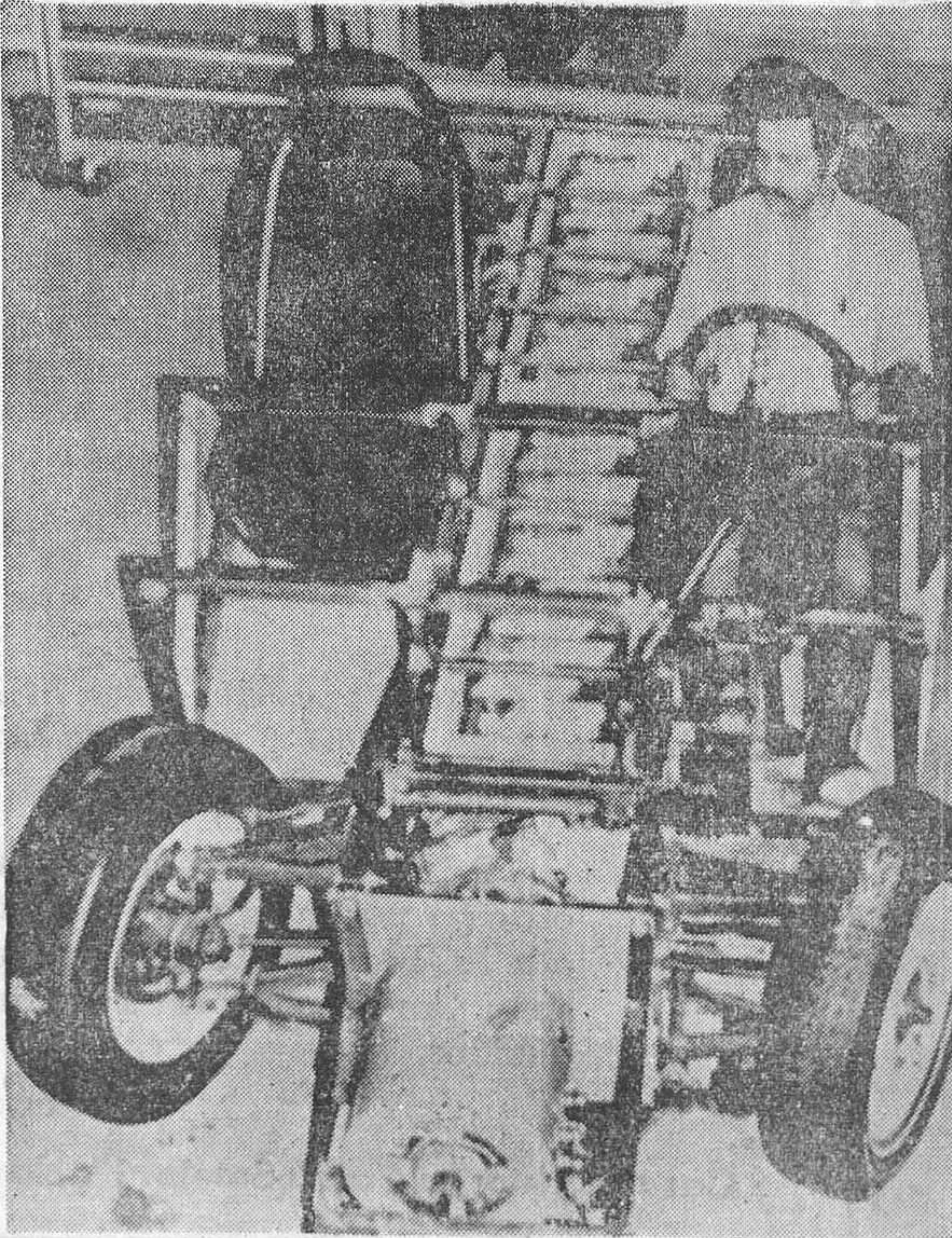
En Atlantic City, un ingeniero, sentado al volante, aparece aquí durante una prueba con el chasis de un "Bedfor" en lo que será un nuevo coche eléctrico, que se planea lanzar al mercado de forma limitada en la próxima primavera
