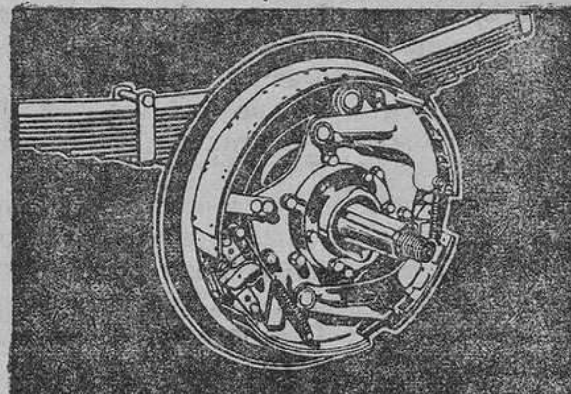
Nuevas ruedas gemelas
