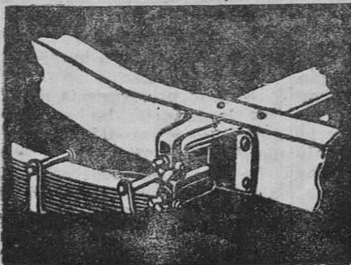
Ballestas semielípticas
