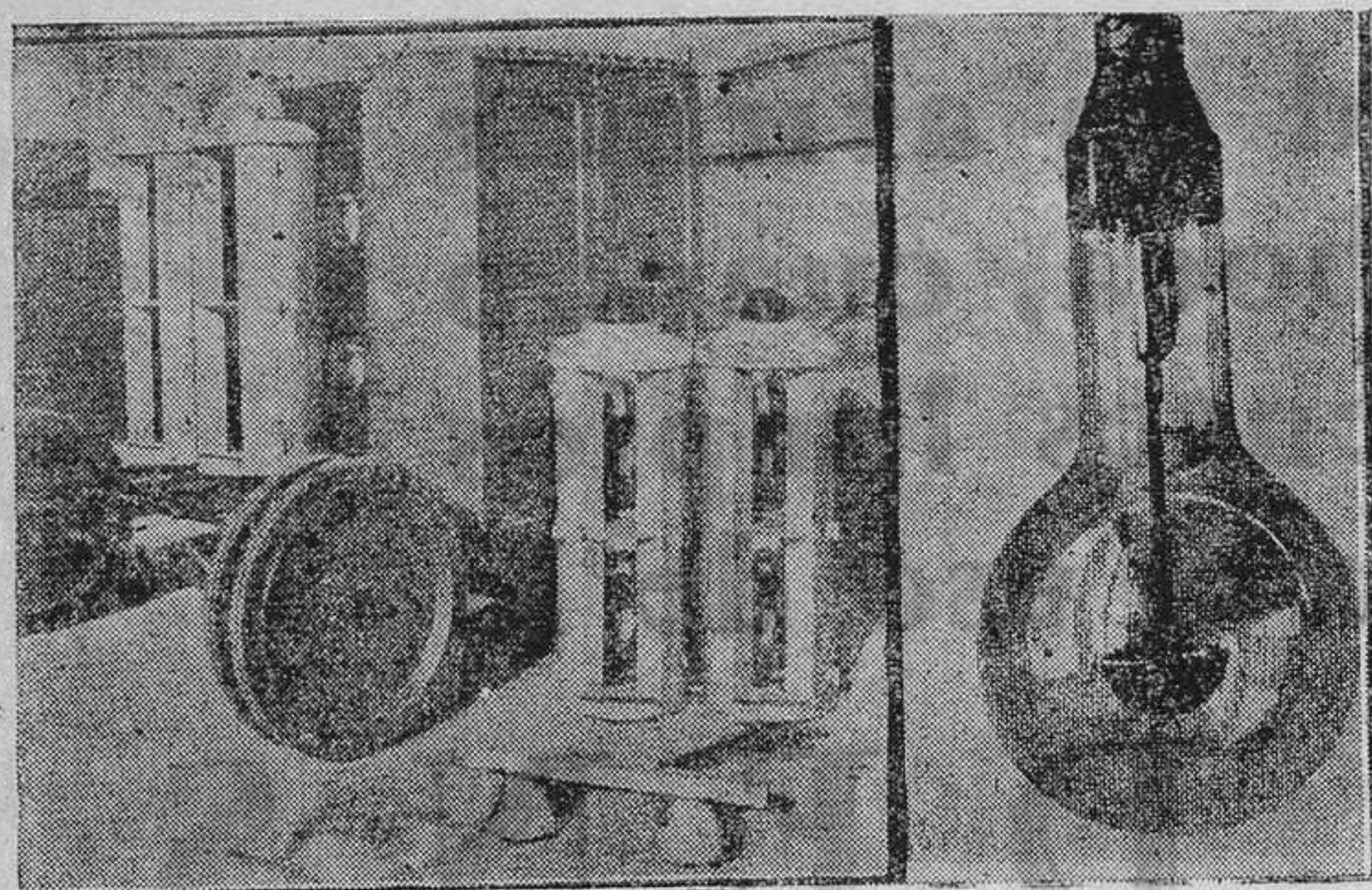
Un carro de proyectores cuádruples montado sobre su correspondiente chasis y éste sobre neumáticos especiales, dispuesto a funcionar. Al lado una lámpara "Brant-Aviation" de 55 voltios 15 amperios que es la utilizada para la iluminación de los aeródromos.
