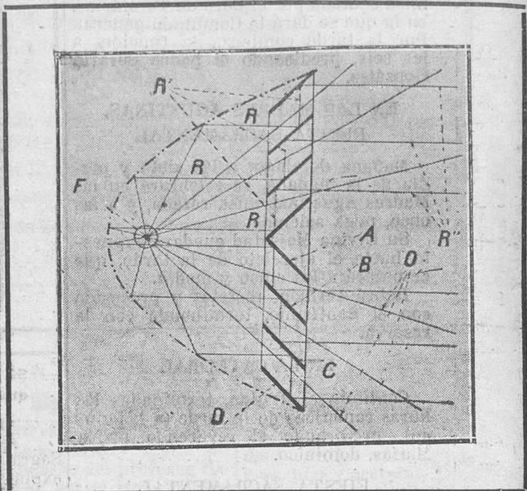
Figura 2.ª—Esquema demostrativo de la disposición general de la pantalla. (Véase el texto)
