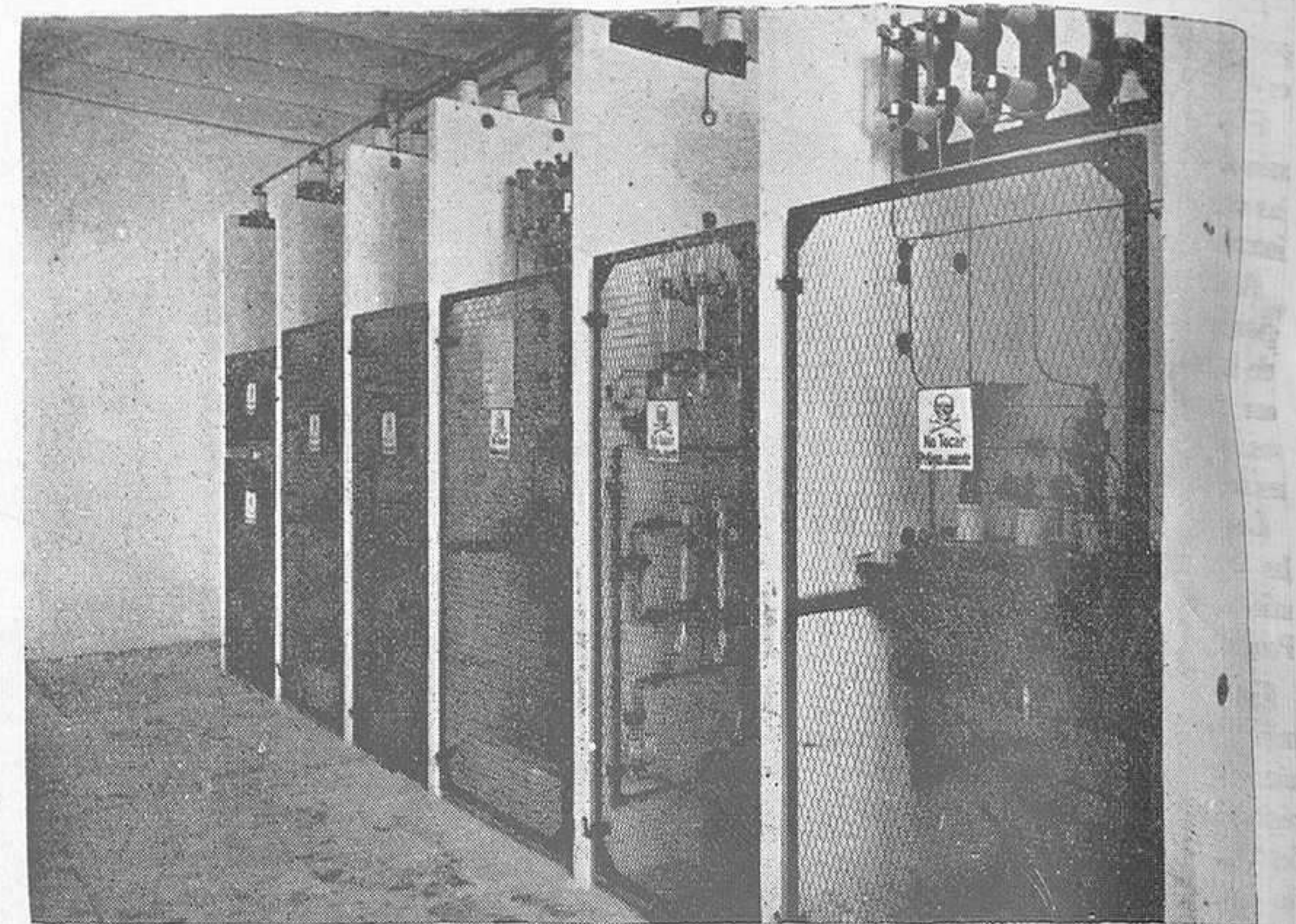
Otro aspecto del cuadro de distribución.
