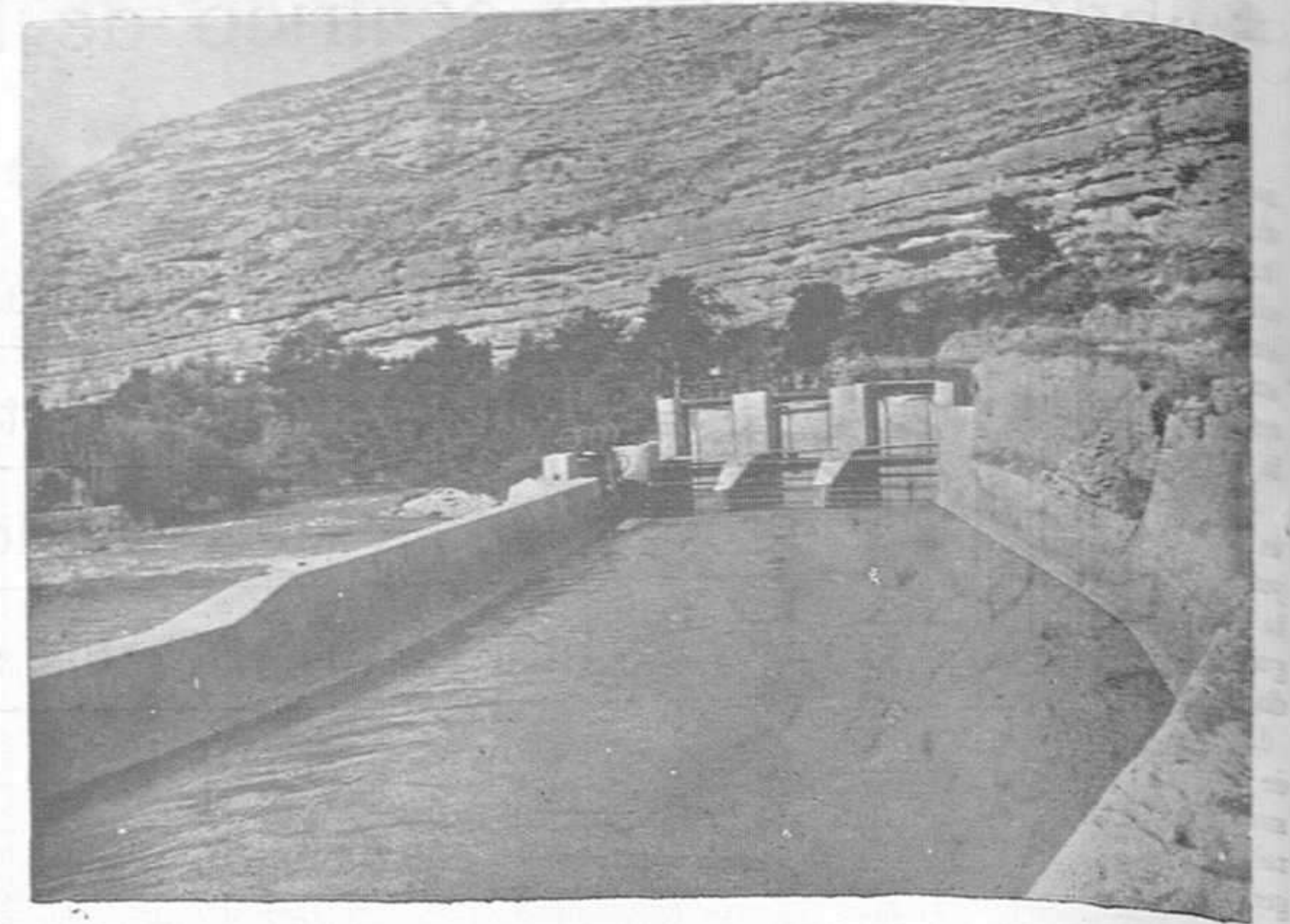
Compuerta de entrada y cuarto de la presa.
