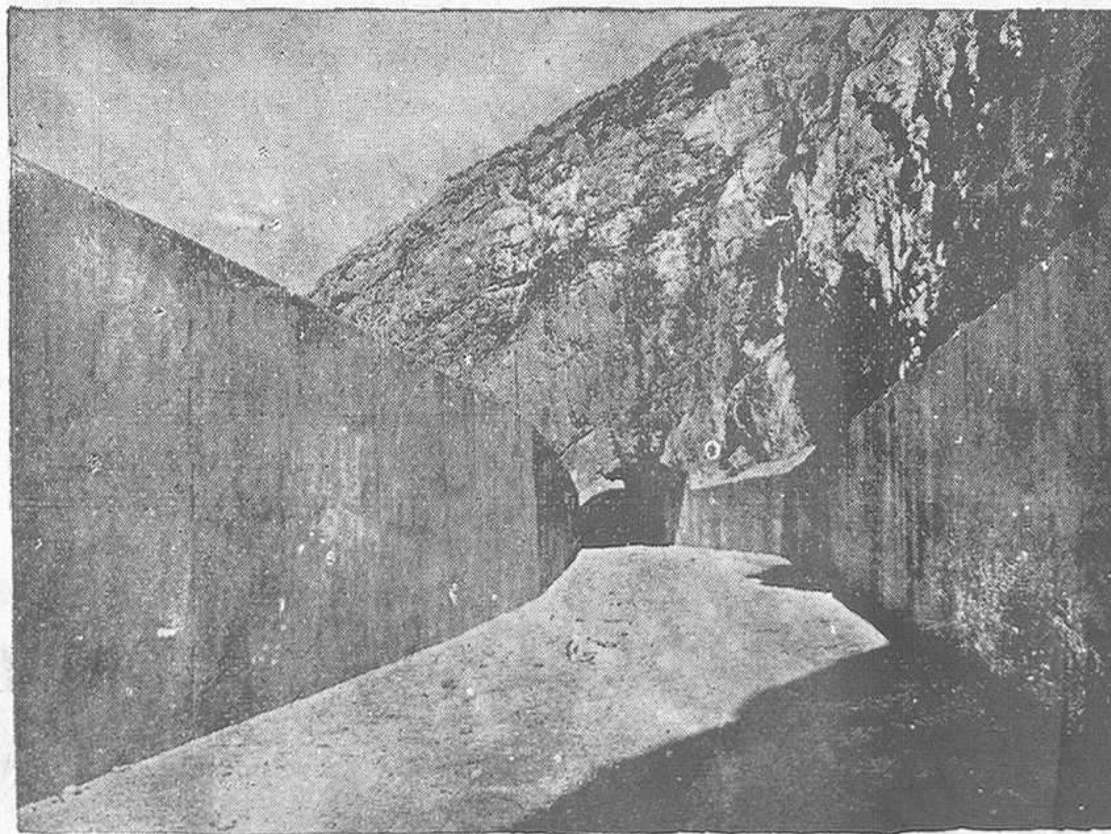
Uno de los trozos del canal y túnel que conduce el agua del Júcar al salto, que sirve para transformar la energía hidráulica en energía eléctrica.
