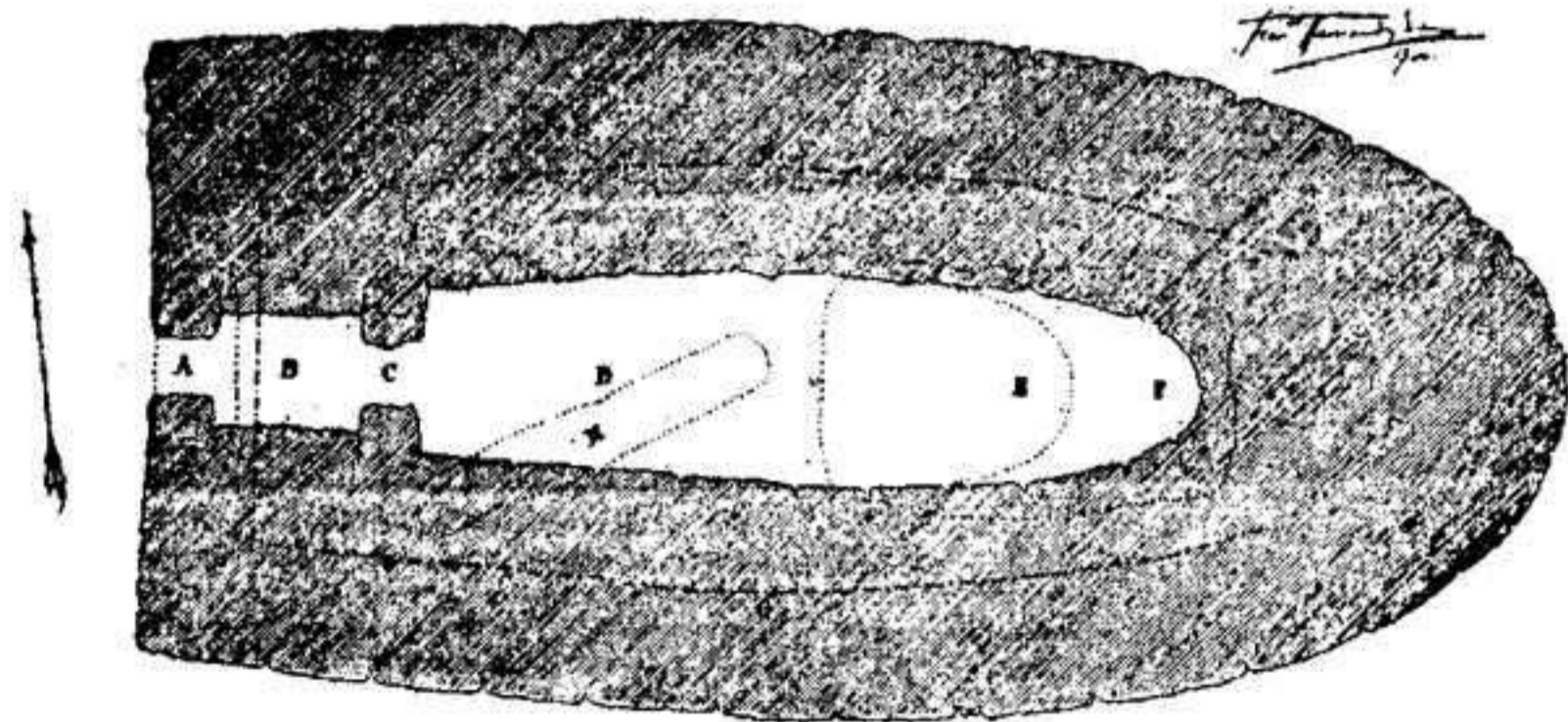
Corte longitudinal y Planta de la NAUETA d' Es Tudons
