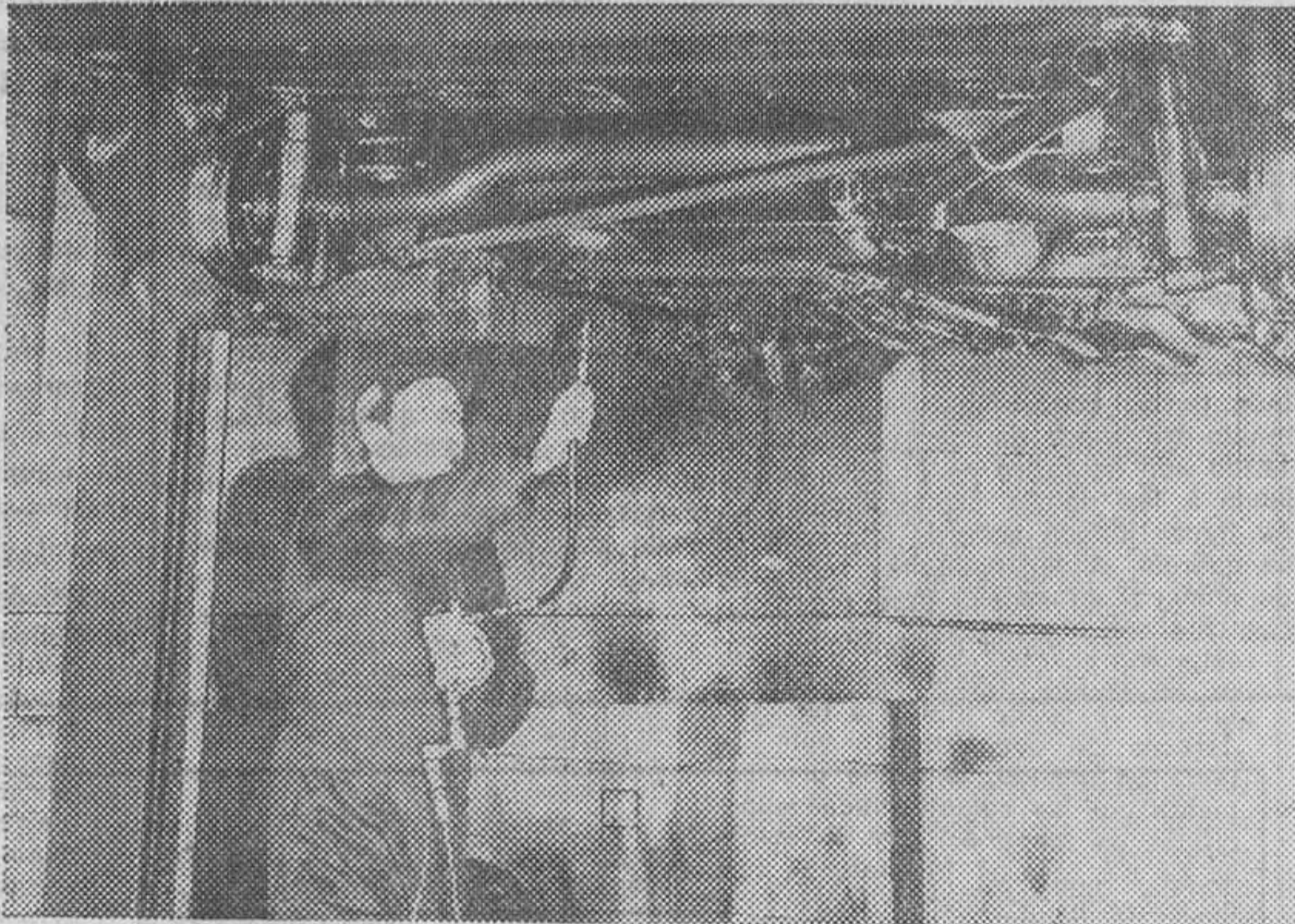
Inyección Dinitrol ML en el faldón del chasis
