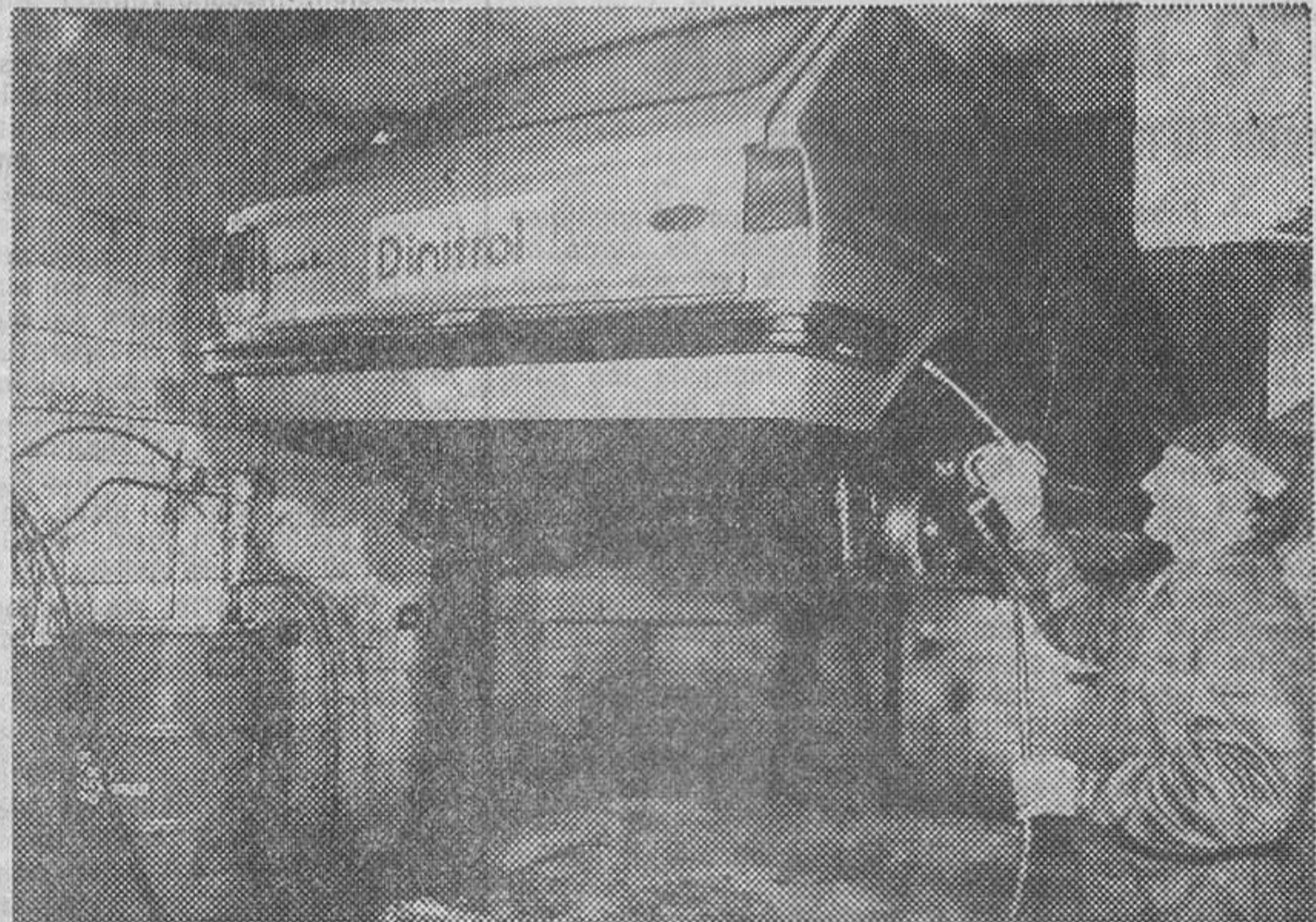
Pulverización de Dinitrol Metallic en el pasarruedas
