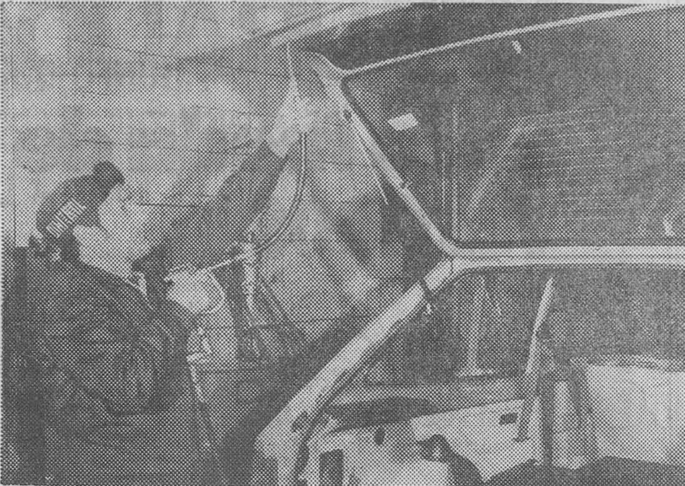
Inyección Dinitrol ML en la tapa portamaletas
