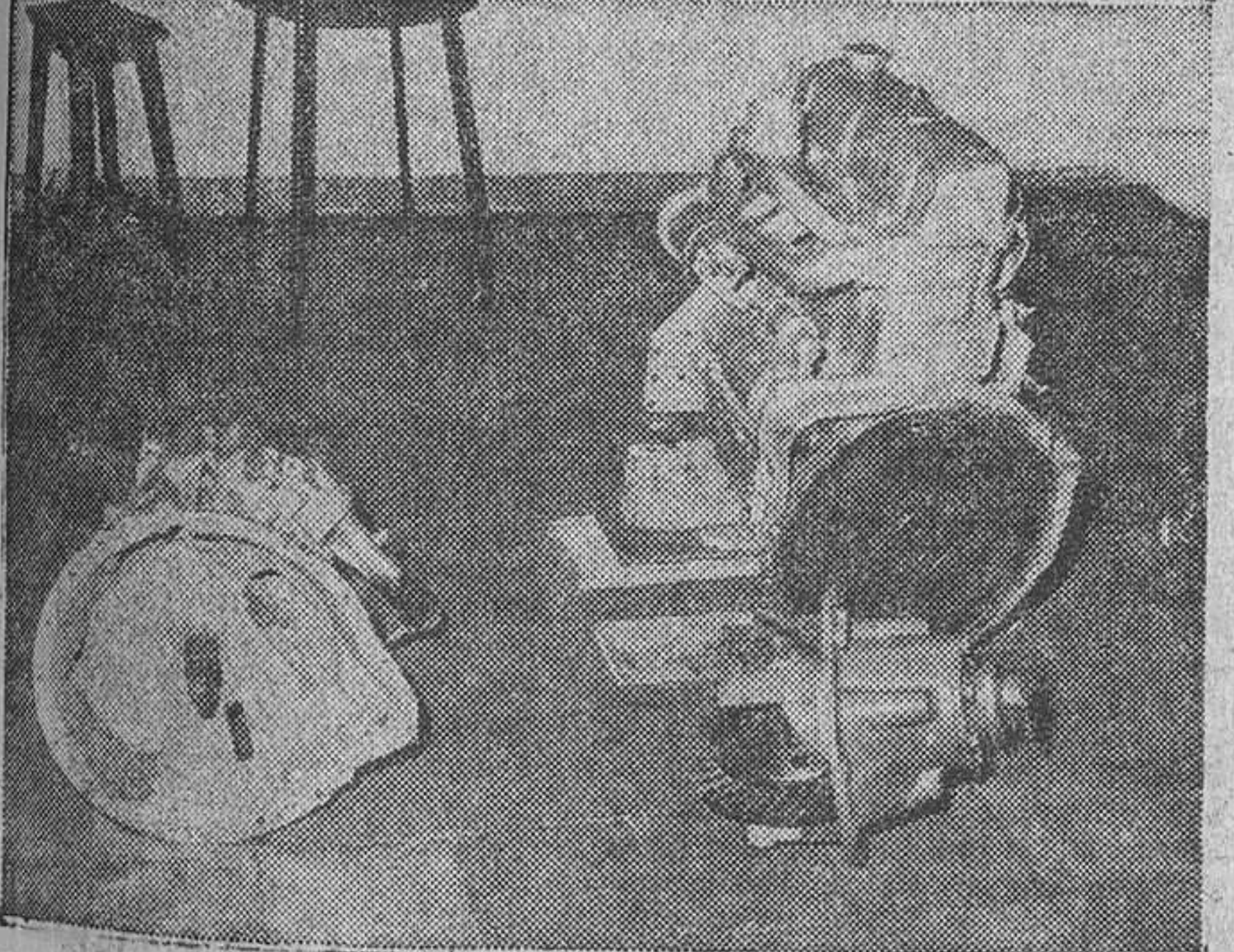
Este es el regalo que ha hecho recientemente Motor Ibérica, S. A. a la Cátedra de Motores de la Escuela de Ingenieros Industriales de Barcelona: un motor EBRO de 70 CV., una caja de cambios de cinco velocidades sincronizadas y un grupo cónico del puente trasero del camión EBRO D-550
