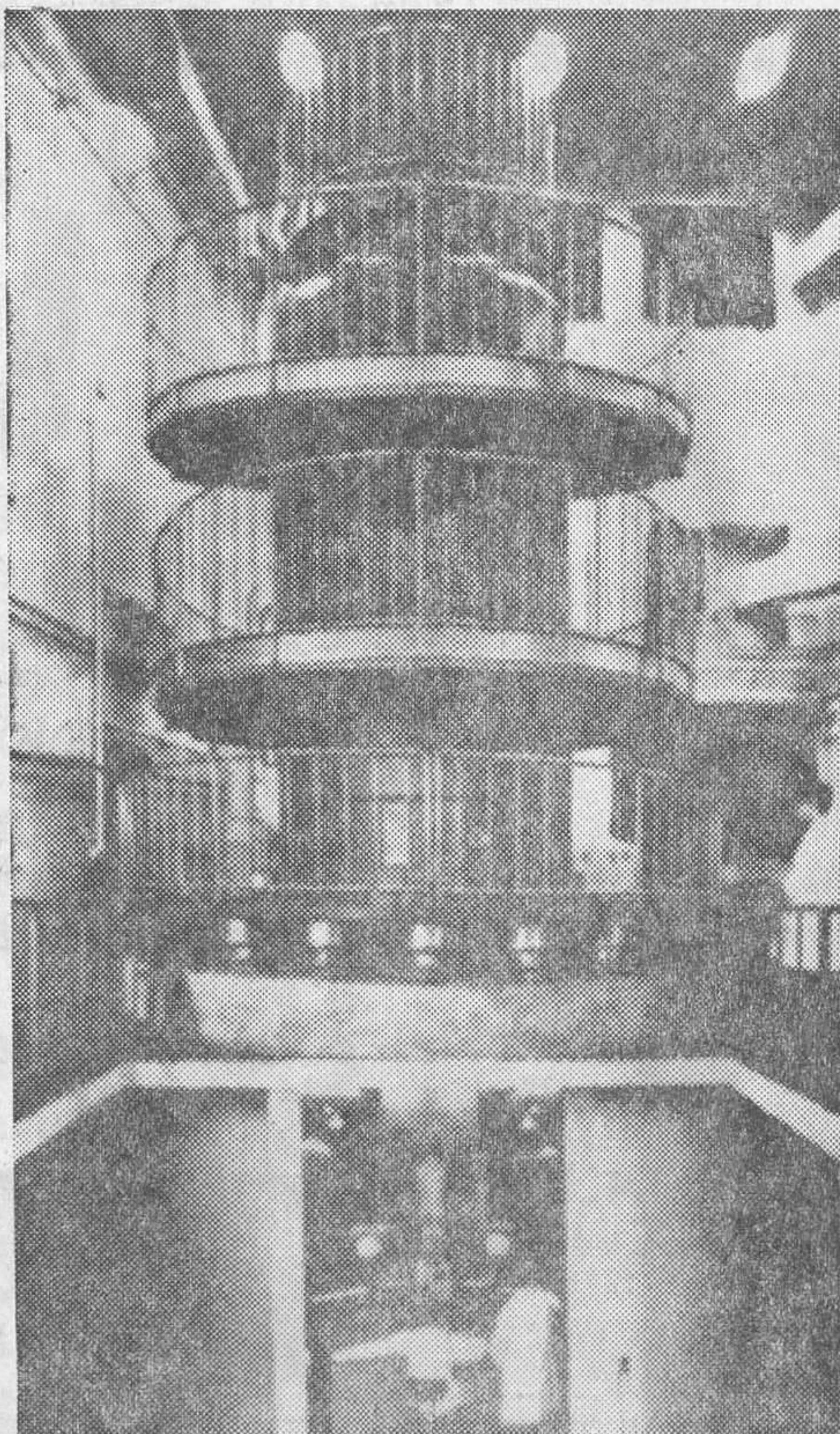
Tokio. — He aquí el microscopio electrónico de tres millones de voltios, construido por la firma japonesa «Hitachi Ltda.». Se trata del más grande del mundo, de estas características. Todos sus instrumentos, montados, tienen una altura aproximada de 15 pisos y un peso de 67 toneladas. — (Telefoto Cifra)
