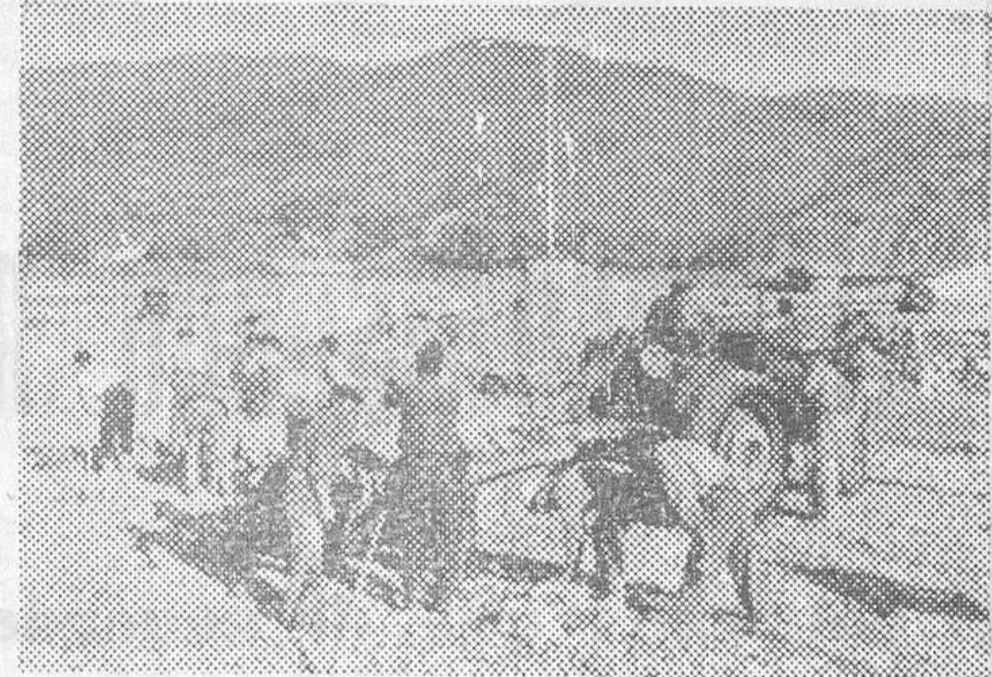
Ya se preparan las pilasstras que habrán de soportar el nuevo puente provisional, cuyas piezas ya están incluso cargadas en los vagones que han de traerlas. Por aquí, dentro de diez días, volverá a pasar el ferrocarril. El río Ripoll, ya casi junto al Besós, habrá perdido la partida
