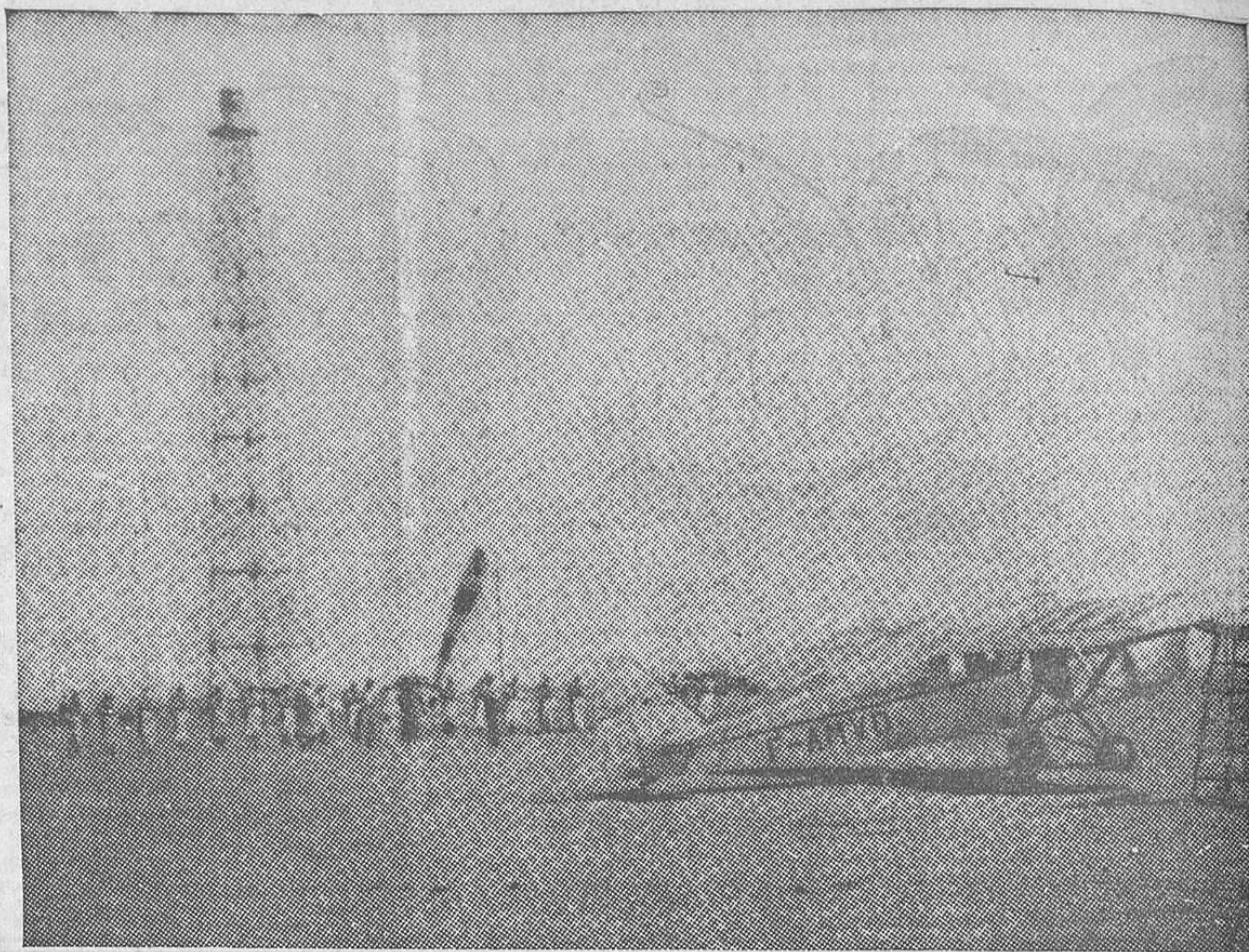
En Vuillemin se ha inaugurado un faro que significa el lazo de unión entre el Africa del Norte y el continente negro. Van a situarse ocho faros, a una distancia de 100 kilómetros el uno del otro, para jalonar el Sahara entre Colomb-Bechar y Gao
