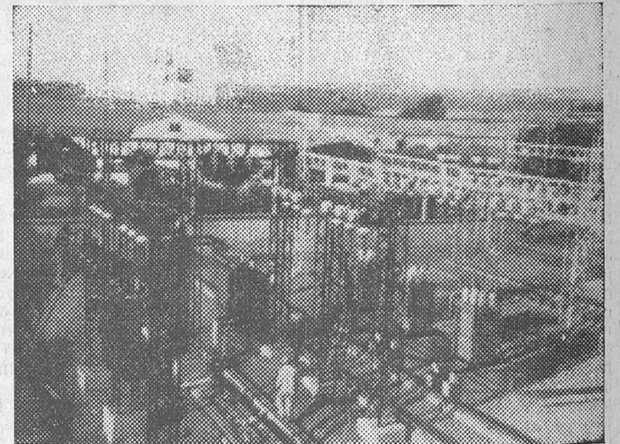
Subestación de Larache.—Lado de 15.000 voltios
