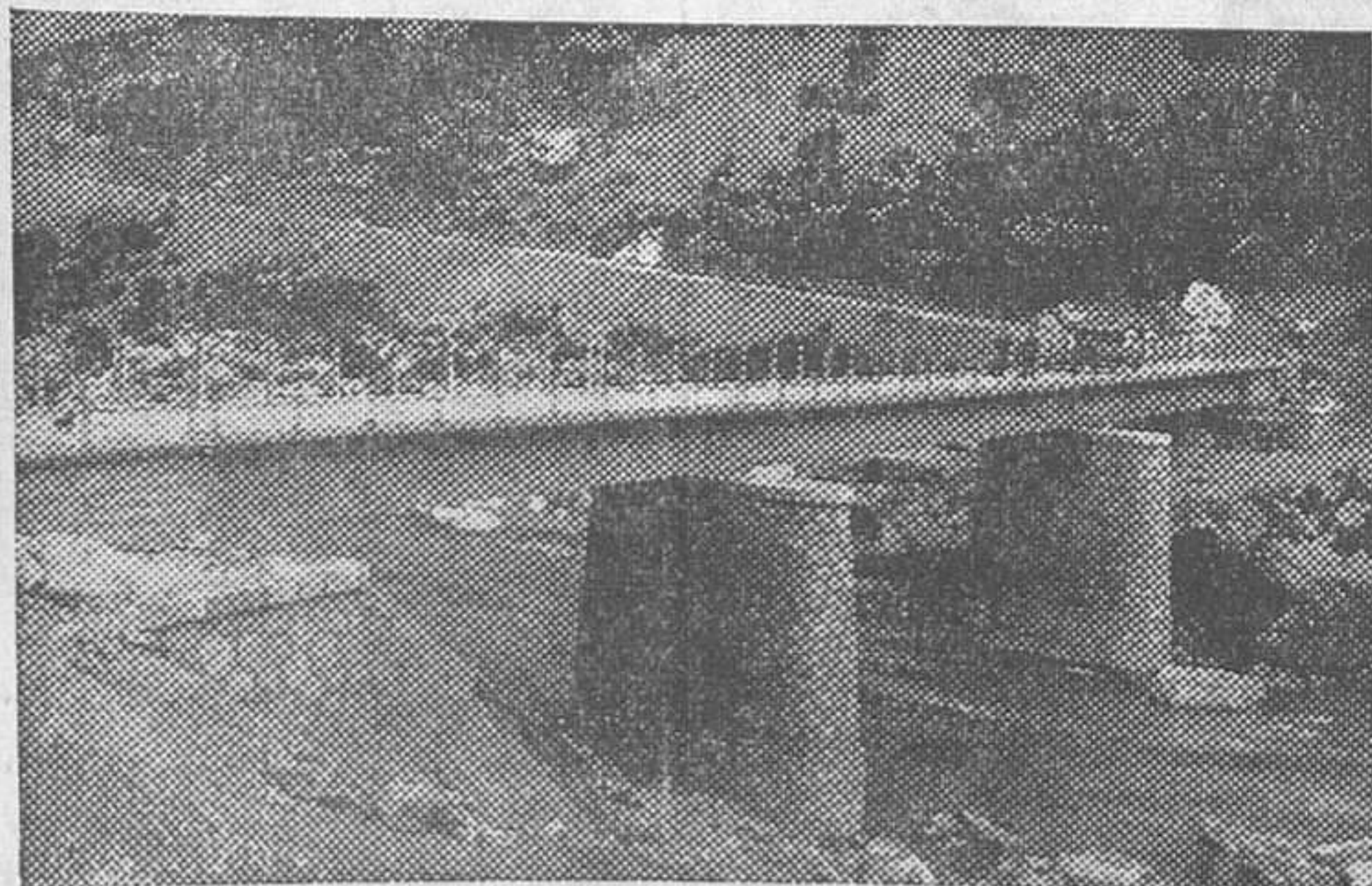
Puente sobre el Lau para apoyo del gran sifón que da paso a las aguas del canal
