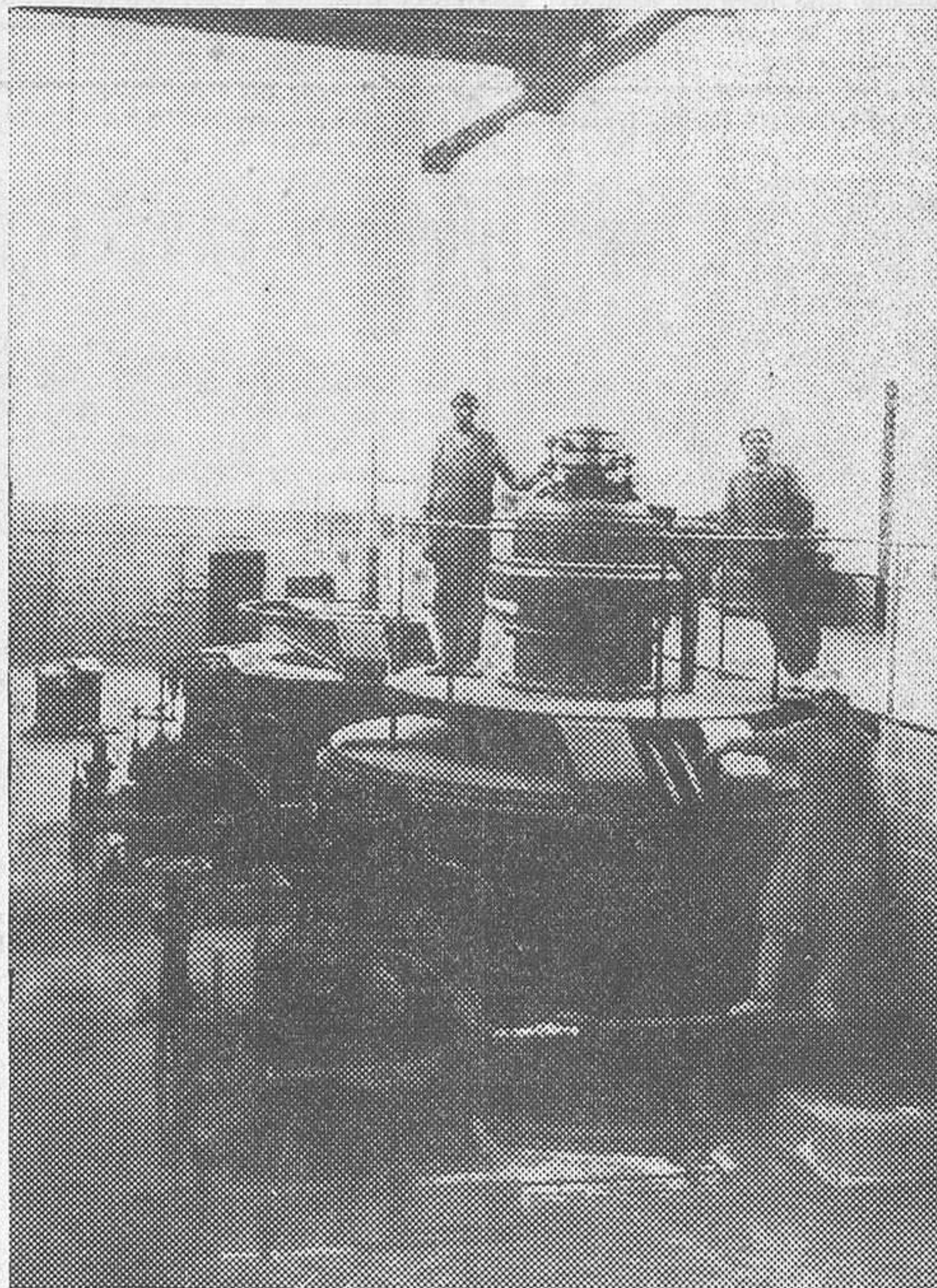
Central río Lau.—Sala de máquinas durante el montaje
