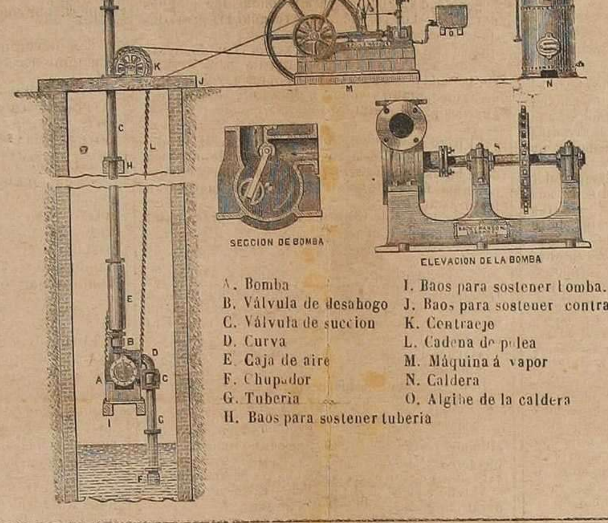
A. Bomba. B. Válvula de desahogo. C. Válvula de succion. D. Curva. E. Caja de aire. F. Chupador. G. Tuberia. H. Baos para sostener tuberia. I. Baos para sostener bomba. J. Baos para sostener contraeje. K. Contraeje. L. Cadena de polea. M. Máquina a vapor. N. Caldera. O. Alighe de la caldera.
