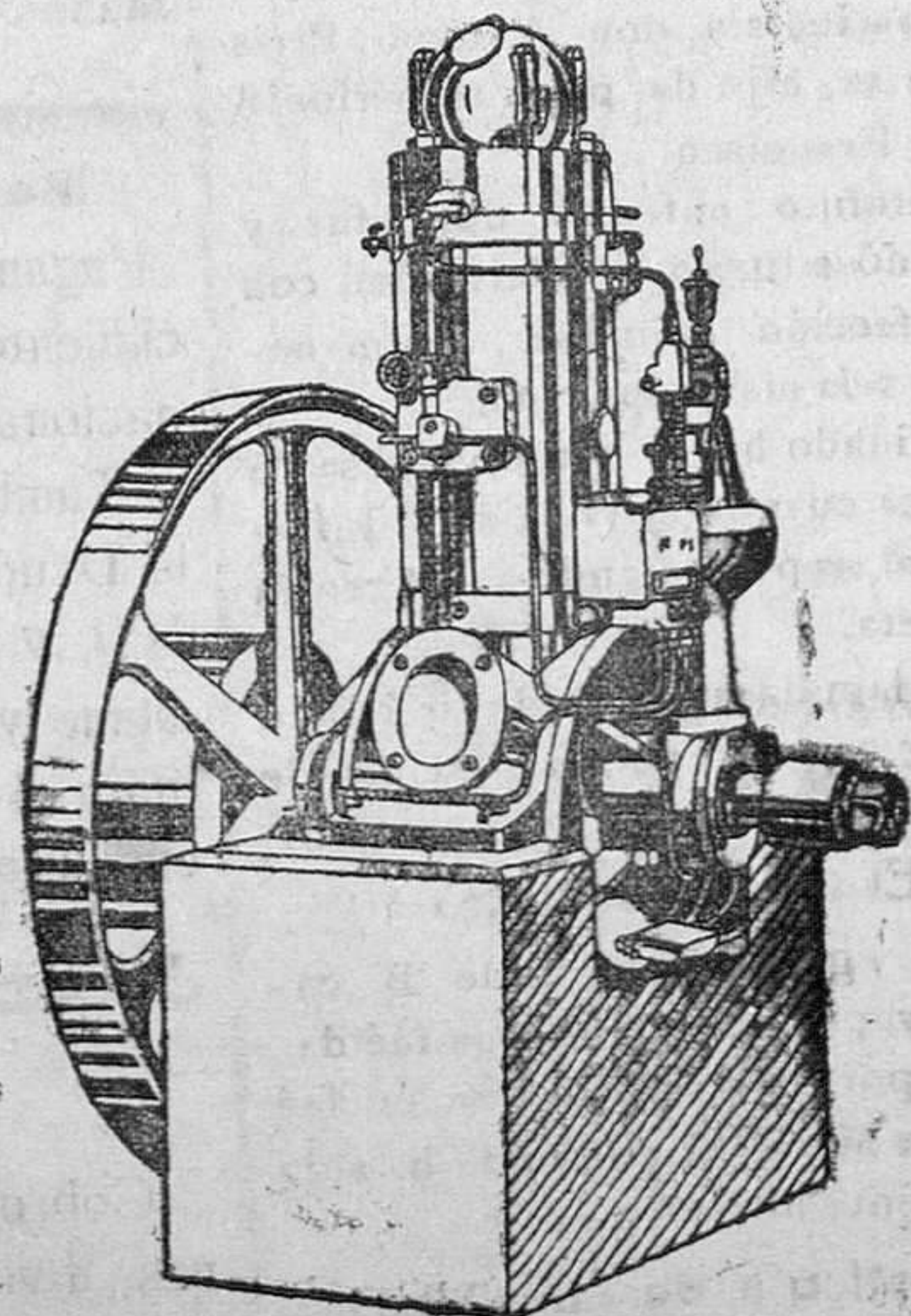
Motor para aceites pesados sin válvulas, sin magneto, adecuada para trilladoras
