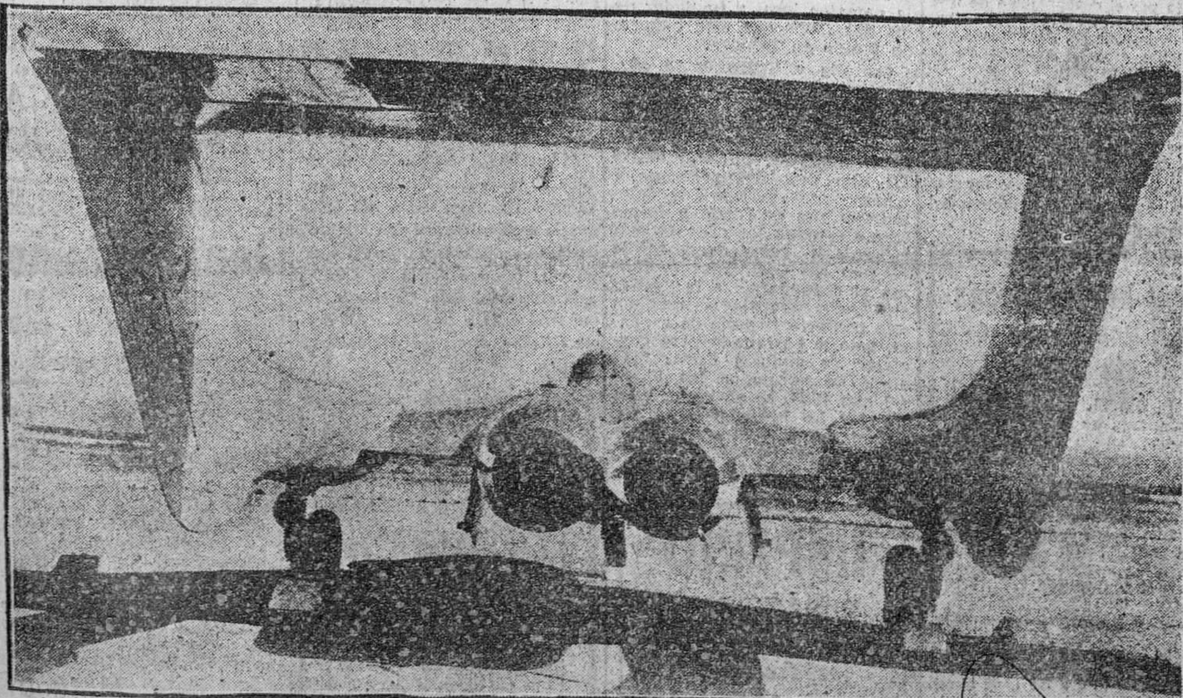
Este es el avión británico «D. H. 119», avión de caza a reacción experimental con destino a la Marina. El aparato, de monstruoso aspecto, ha sido fotografiado durante la exhibición y prueba en el festival de Farborough.
