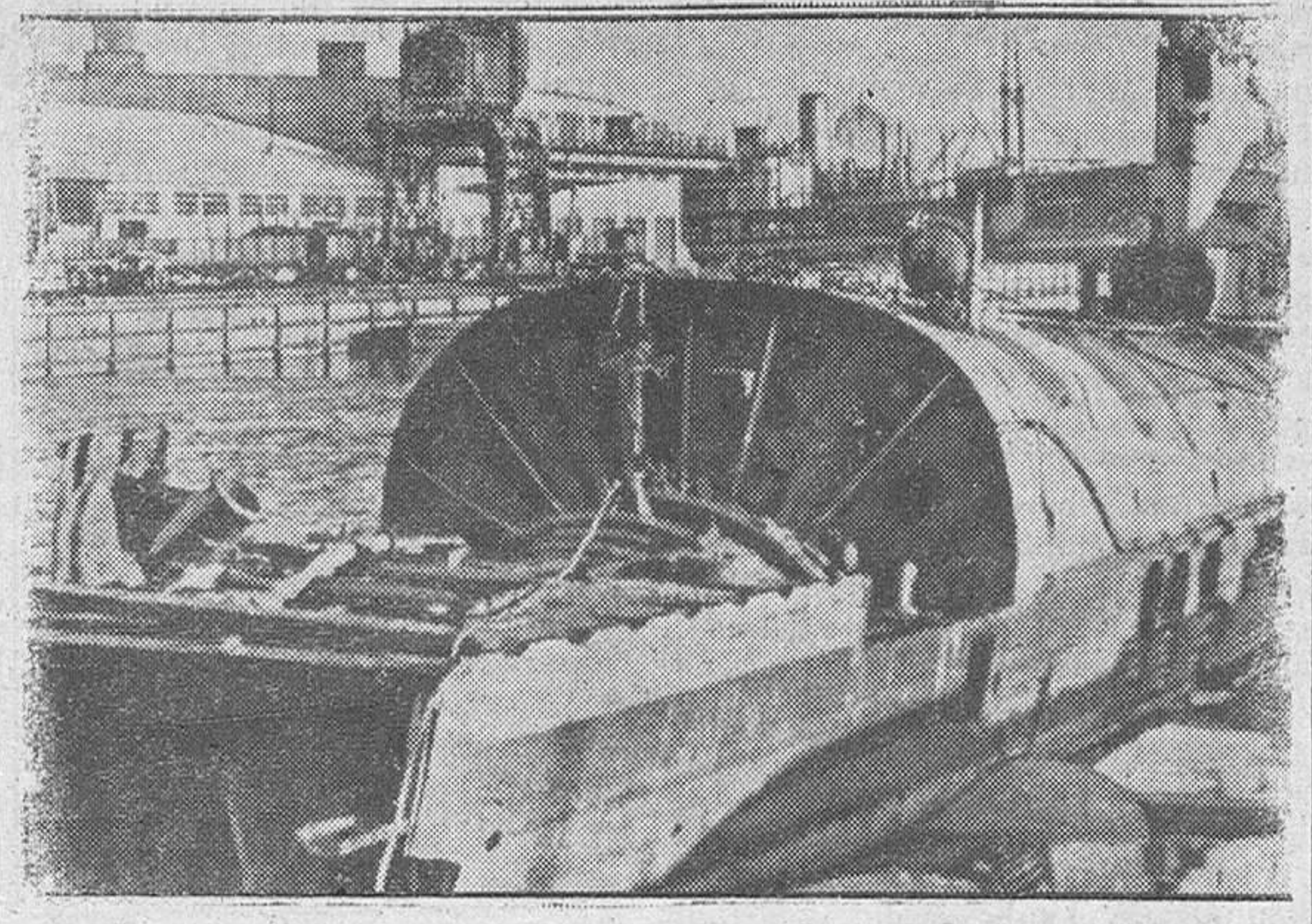
El submarino sueco «Ulven» que fué hundido en abril de 1943 con sus 36 tripulantes, ha sido recientemente sacado a flote en el puerto de Götterburg
