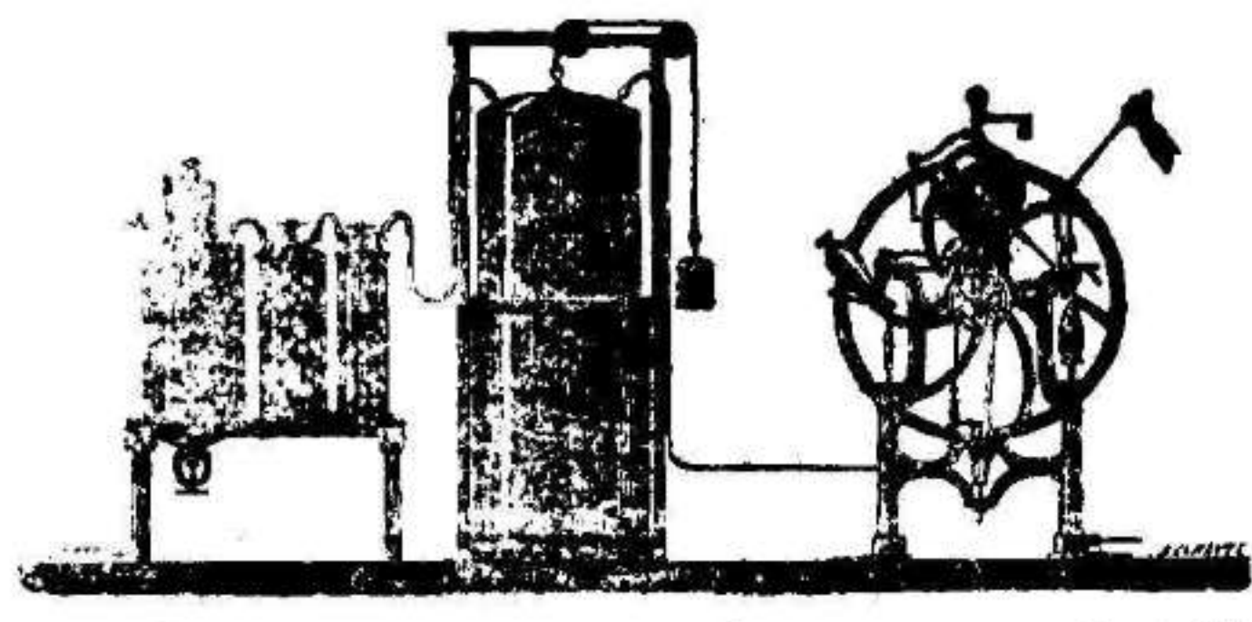
Aparato para gaseosa, continuo con embotella- doras unidas.
