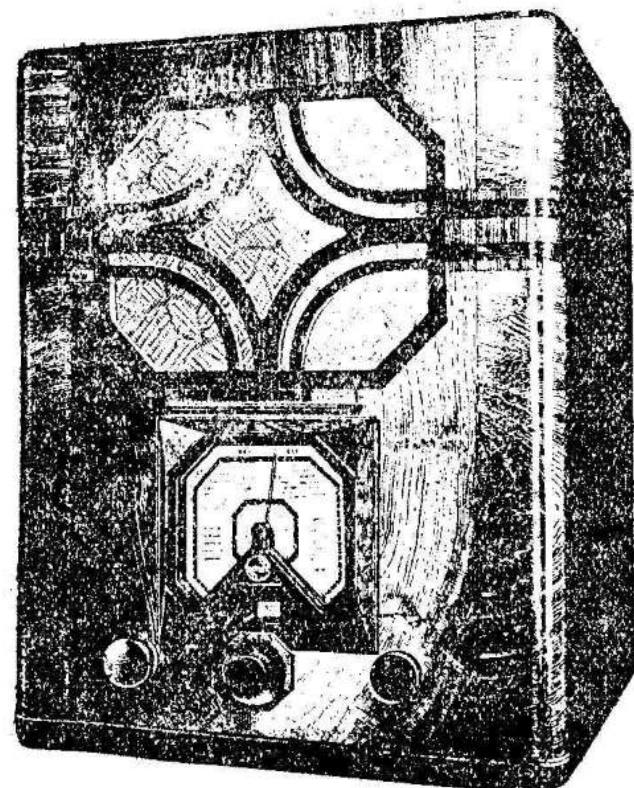
638 A.—Receptor de primera categoría, cuatro circuitos a SUPERINDUCTANCIA, corriente alterna, todos voltajes, ondas cortas y largas, antena incorporada, con escala de emisoras intercambiable. Precio: 845 ptas.
