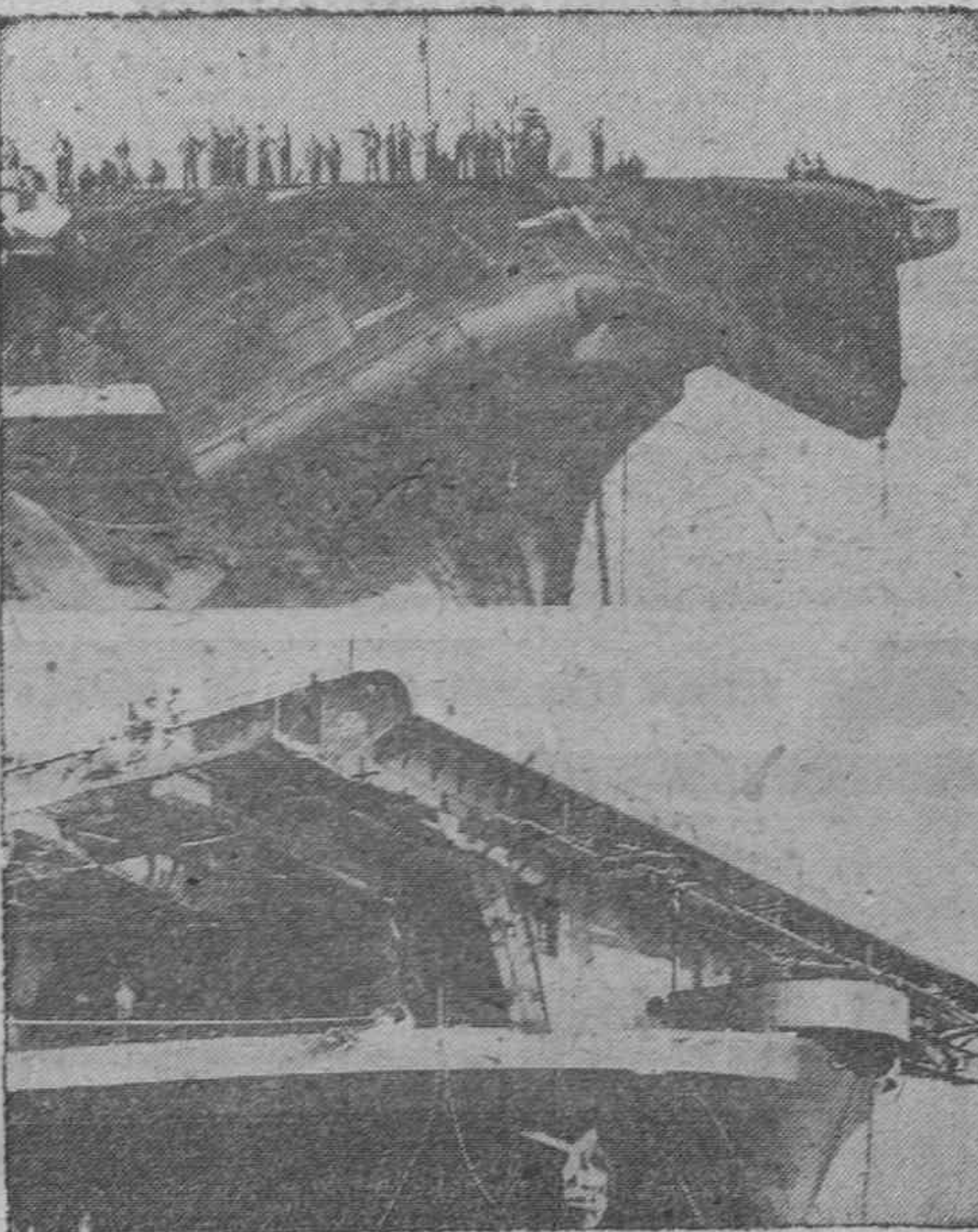
Después de las averías sufridas por un avión en el Pacífico, el portaaviones "Nemiglon" éste quedó totalmente reparado, en el mar, en menos de dos semanas. La foto de arriba nos muestra al portaaviones antes de la reparación.
