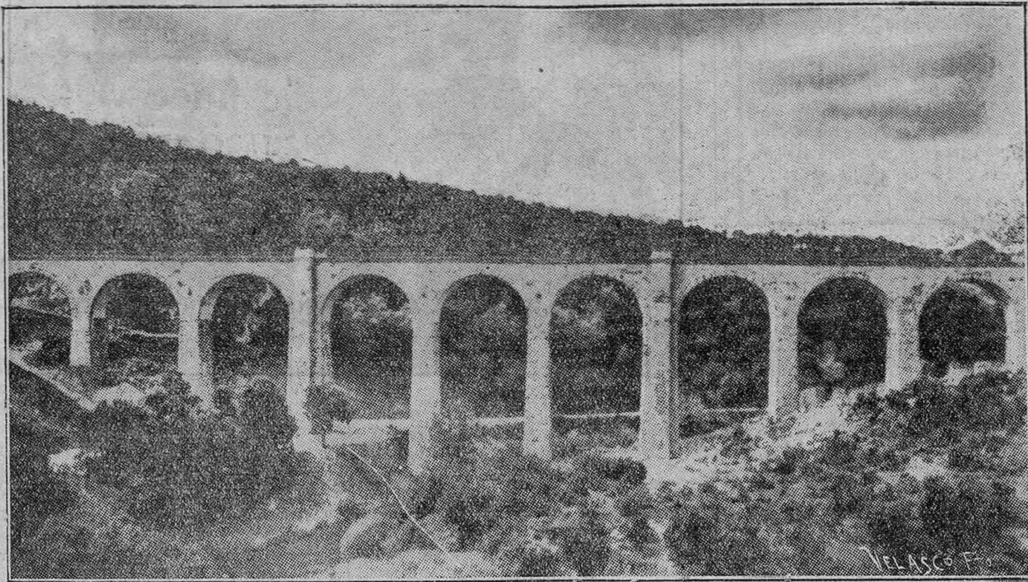
EL VIADUCTO DE ARQUIJAS
