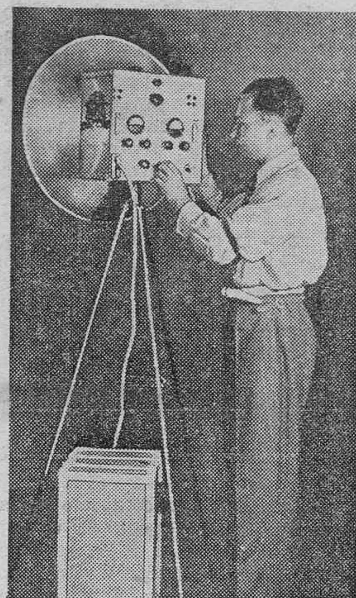
Un receptor para el nuevo sistema de radio, llamado de ondas decimétricas, inventado por la Telefunken...
