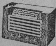
MARCONI (Modelo P-50) 5 lámparas múltiples. 3 márgenes de onda. Altavoz de imán permanente. Control de tono progresivo. Mueble madera con apliques baquelita. Precio v. p. 2.315' - Ptas.
