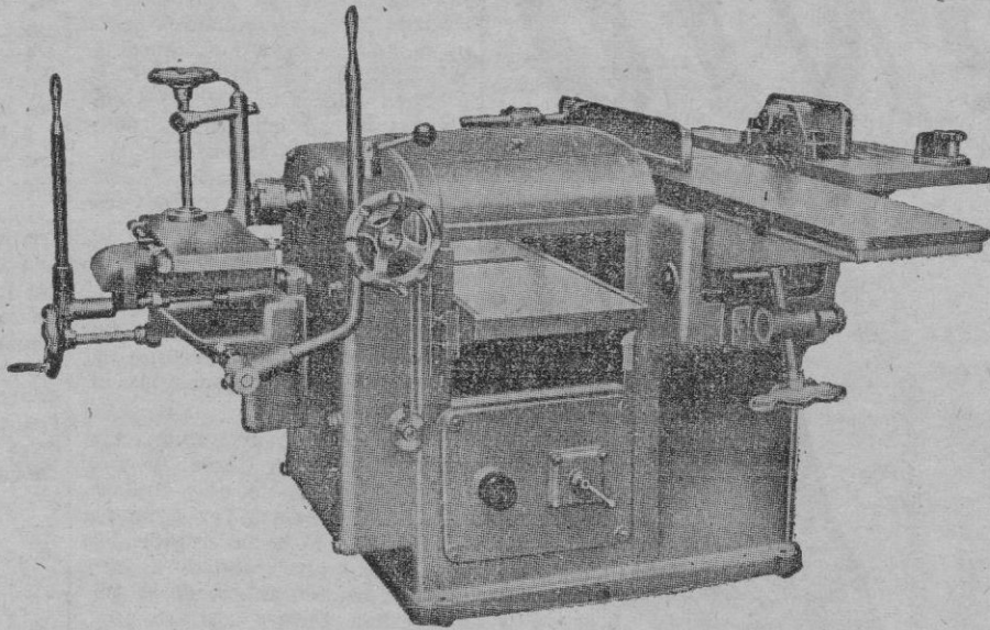
Modelo "Diana", máquina combinada universal con tupi vertical y motores eléctricos acoplados.
