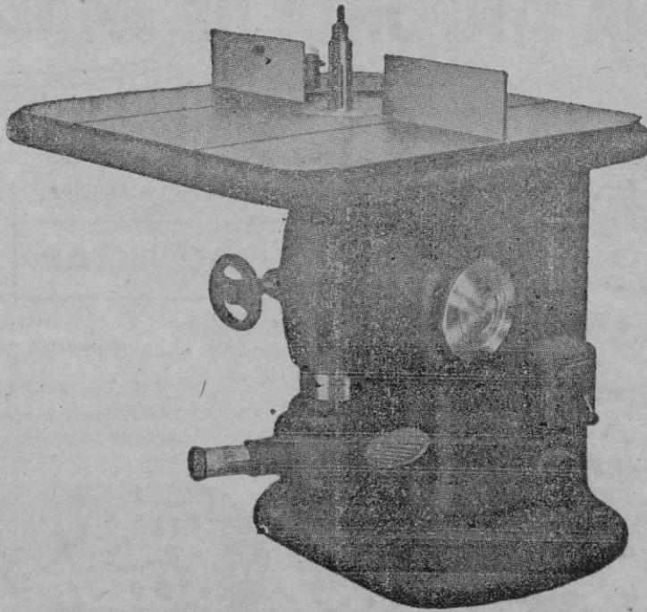
Modelo "Vaprisa", tupi vertical para moldurar con motor acoplado de dos velocidades
