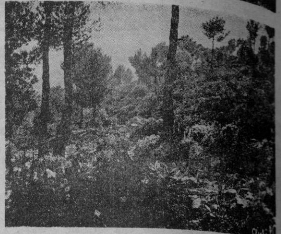
El monte de Benifaldó, del término municipal de Escorca, perteneciente del Patrimonio Forestal del Estado, en periodo de repoblación natural.
