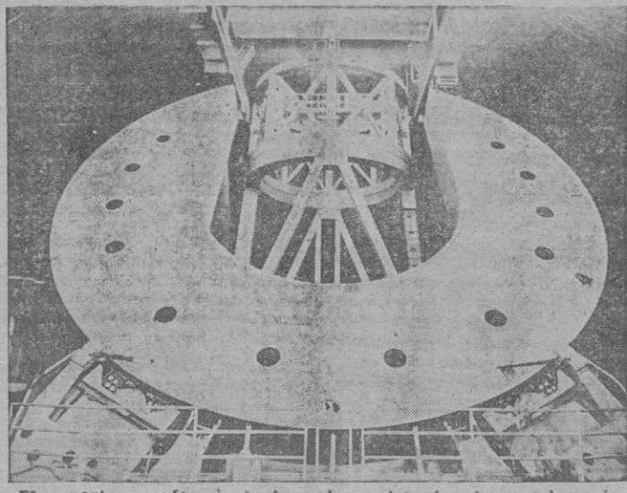
El soporte, en forma de herradura, del gigantesco telescopio
