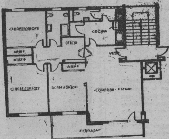
TIPO "B" superficie 103.72 m²
