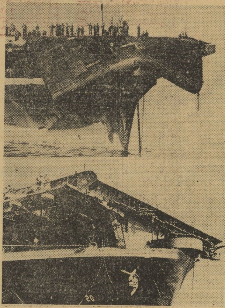
Un violentísimo tifón ha averiado la cubierta de vuelo del portaaviones norteamericano "Bennington". Arriba, antes de la reparación; abajo, después de los trabajos. — (Foto Sena)
