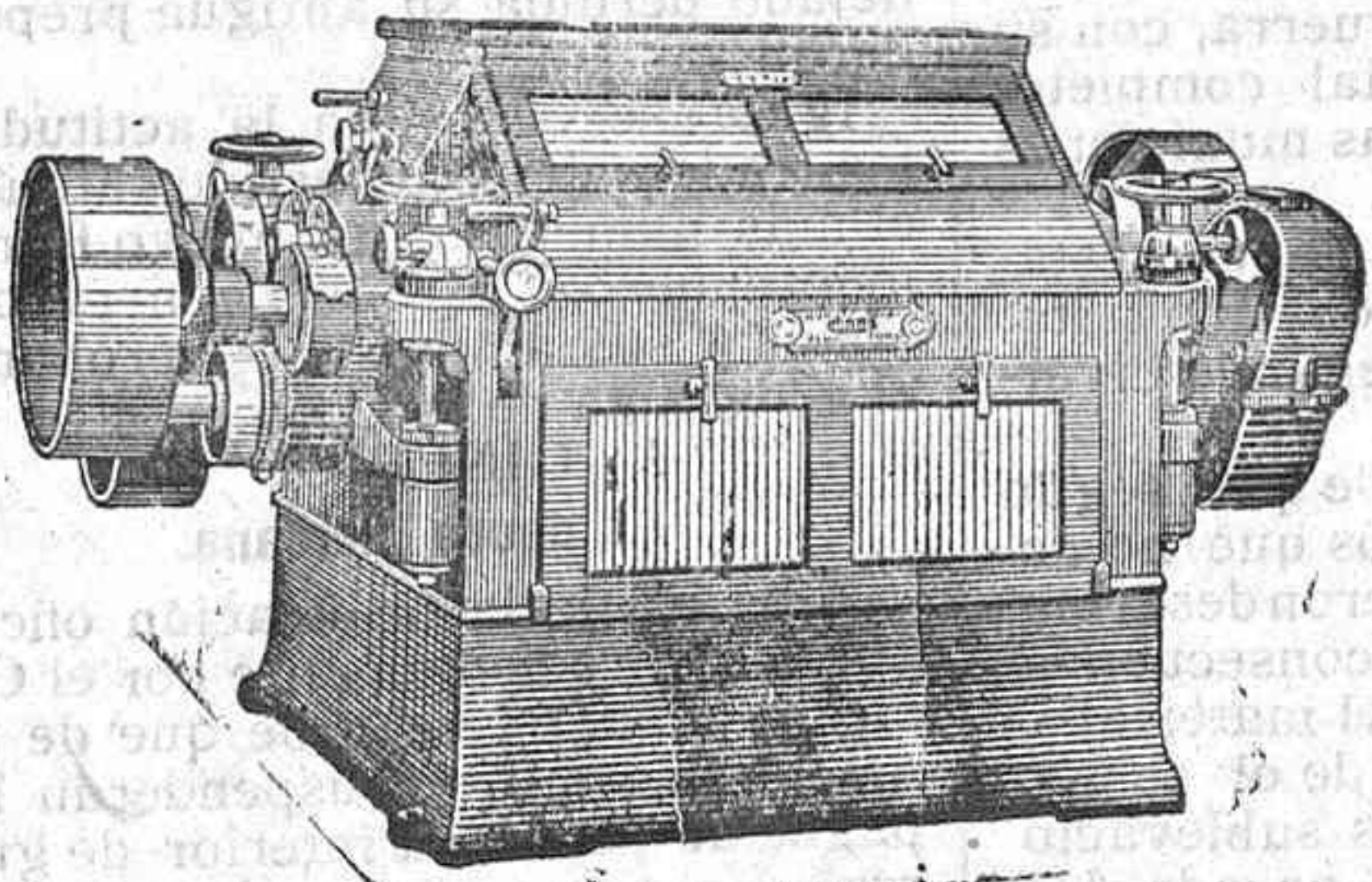
Molino modelo DD de cuatro cilindros. Privilégio BÜHLER
